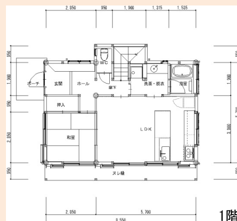
＜展示住宅・生活体験施設の平面図＞
