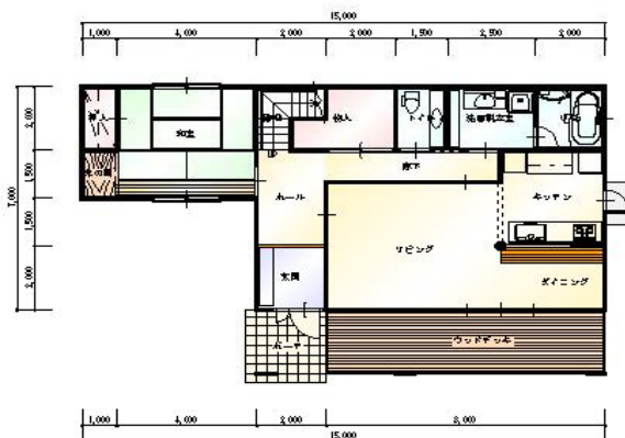
1階 平面図 S:1/100
