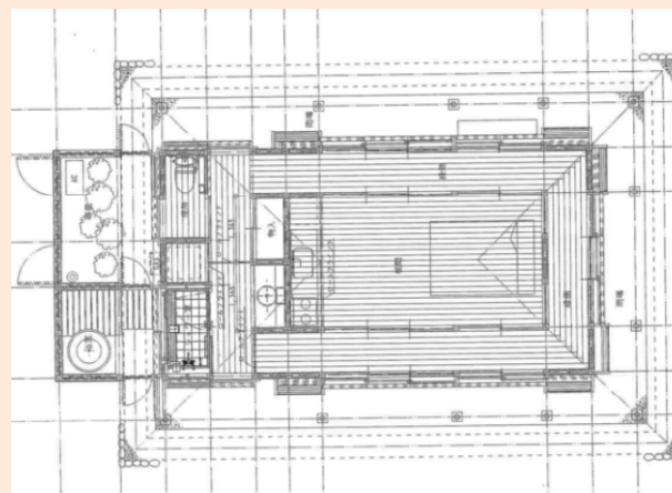
＜展示住宅・生活体験施設の平面図＞
