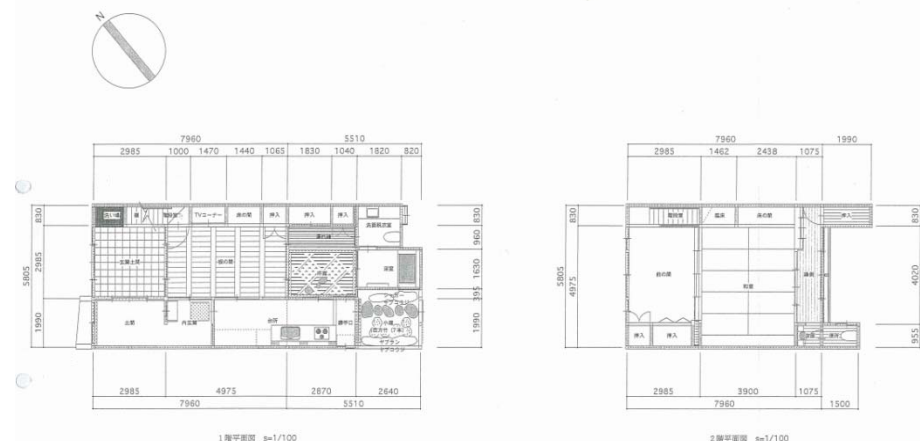
＜展示住宅・生活体験施設の平面図＞
