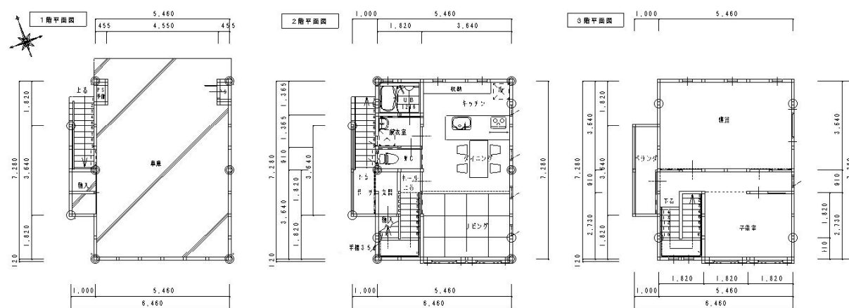
<展示住宅・生活体験施設の平面図>
