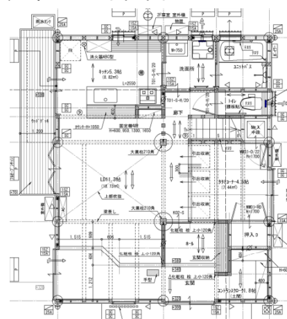
<展示住宅の平面図>
