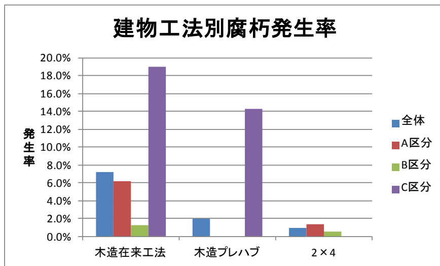
図 6-1 建物工法別腐朽発生率
