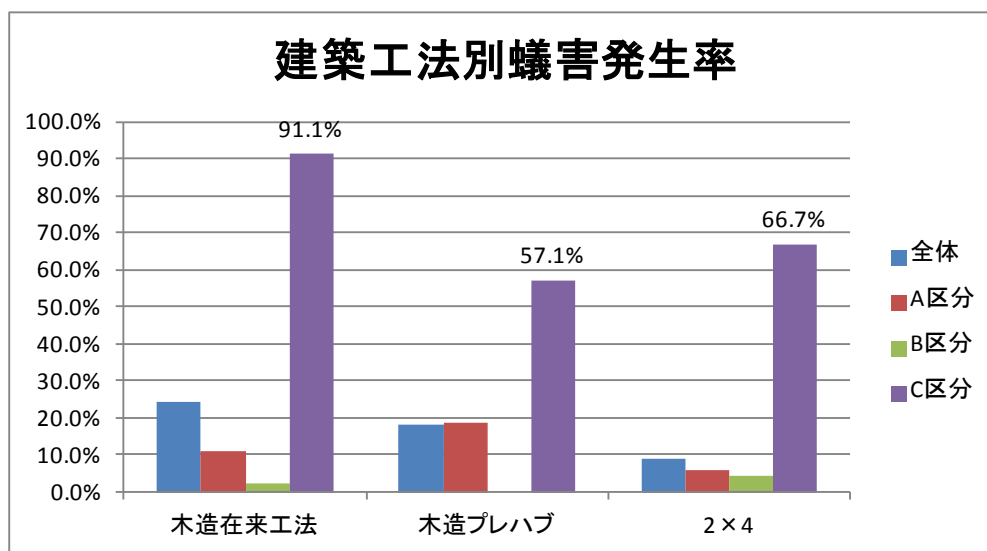
図 5-1 建物工法別蟻害発生率
