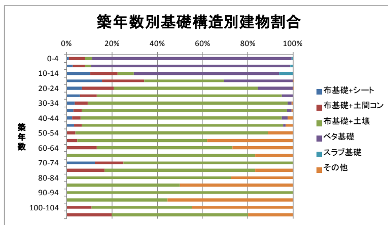
図 3-6 築年数別基礎構造別建物割合
