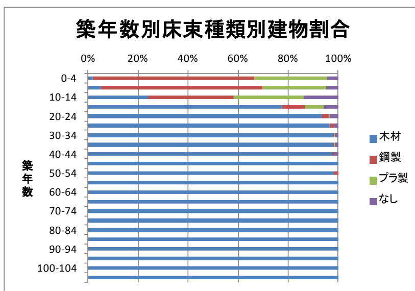
図 3-10 築年数別床束種類別建物割合
