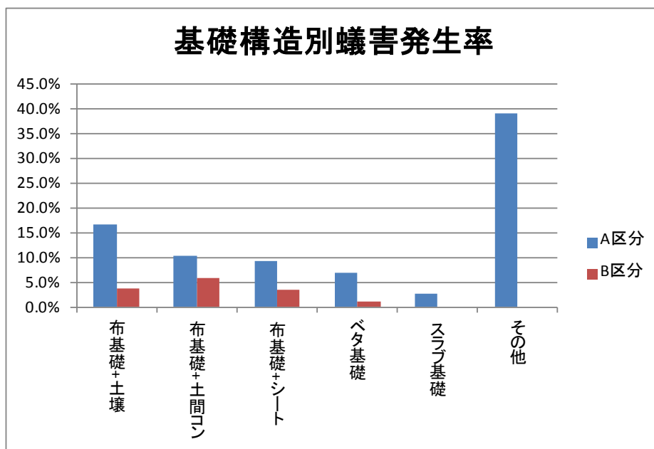
図 5-3 基礎構造別蟻害発生率
