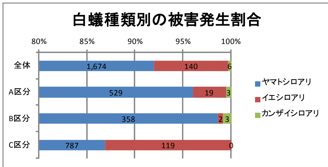
図 4-9 データ区分別蟻害発生棟数に対する白蟻種別の発生割合
