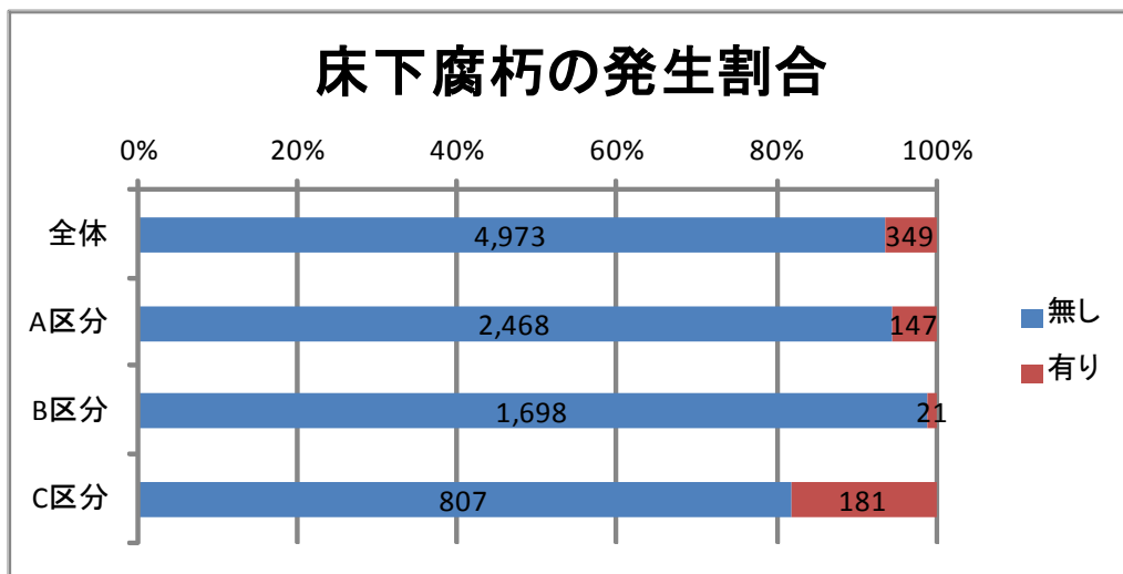
図 4-3 データ区分別床下腐朽の発生割合
