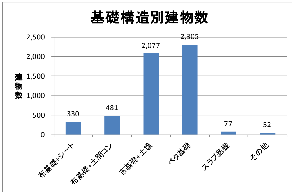
図 3-5 基礎構造別建物数
