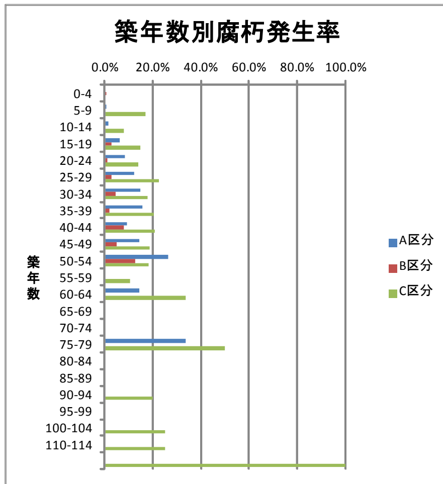
図 6-2 築年数別腐朽発生率
