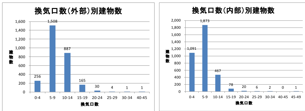
図 3-13 床下換気口数別建物数（左：外周 右：内部）
