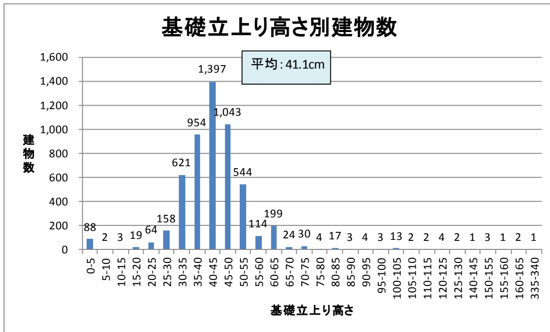
図 3-14 基礎立ち上がり高さ別建物数
