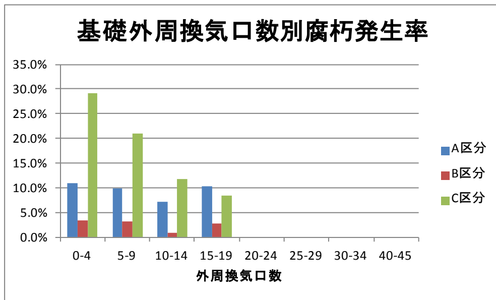
図 6-5 基礎外周換気口数別腐朽発生率
