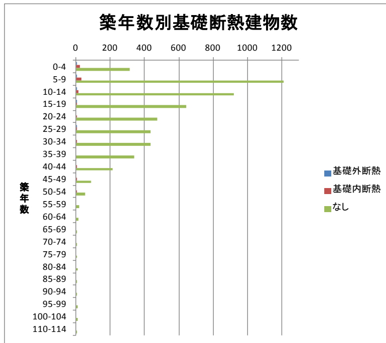
図 3-8 築年数別基礎断熱種別建物数
