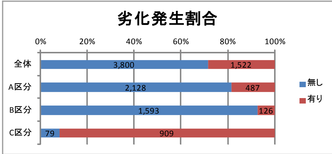
図 4-1 データ区分別生物劣化発生割合
