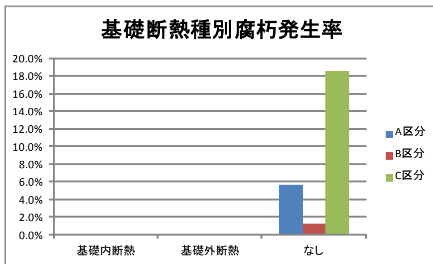
図 6-4 基礎断熱種別腐朽発生率
