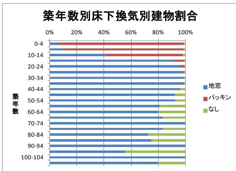
図 3-12 築年数別床下換気種類別建物割合
