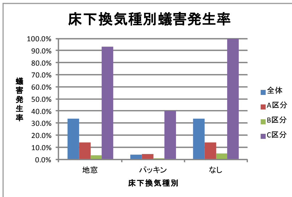
図 5-5 床下換気種別蟻害発生率
