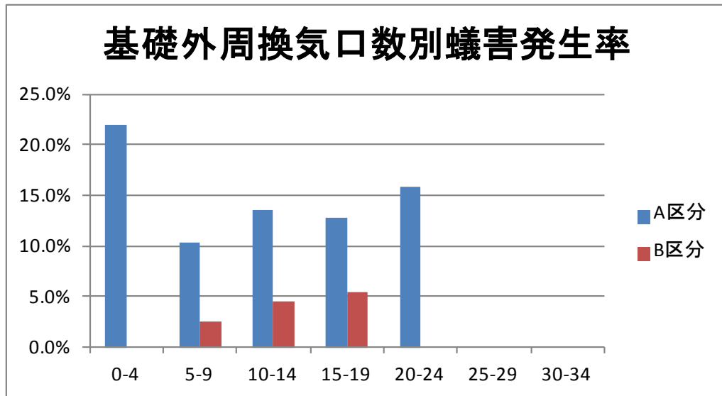
図 5-6 基礎外周換気口数別蟻害発生率
