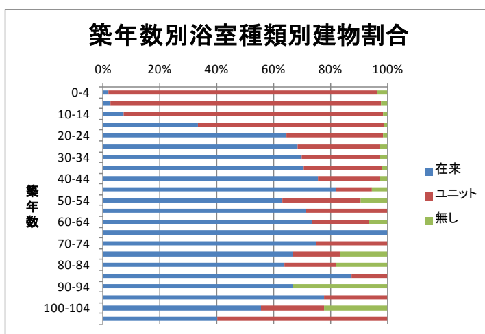
図 3-16 築年数別浴室種類別建物割合
