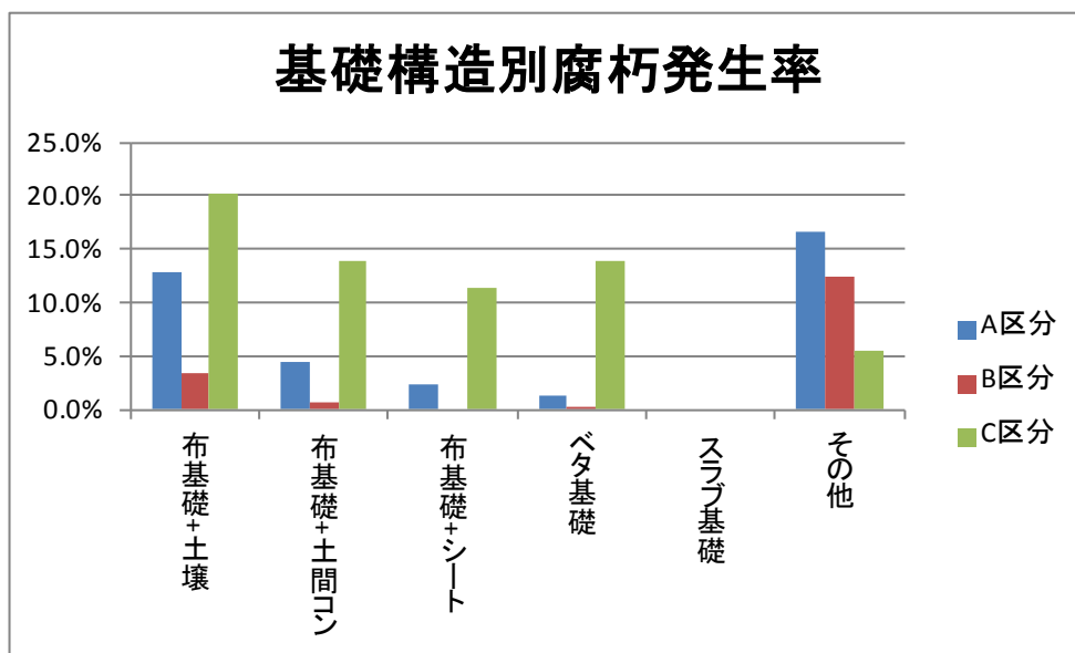
図 6-3 基礎構造別腐朽発生率
