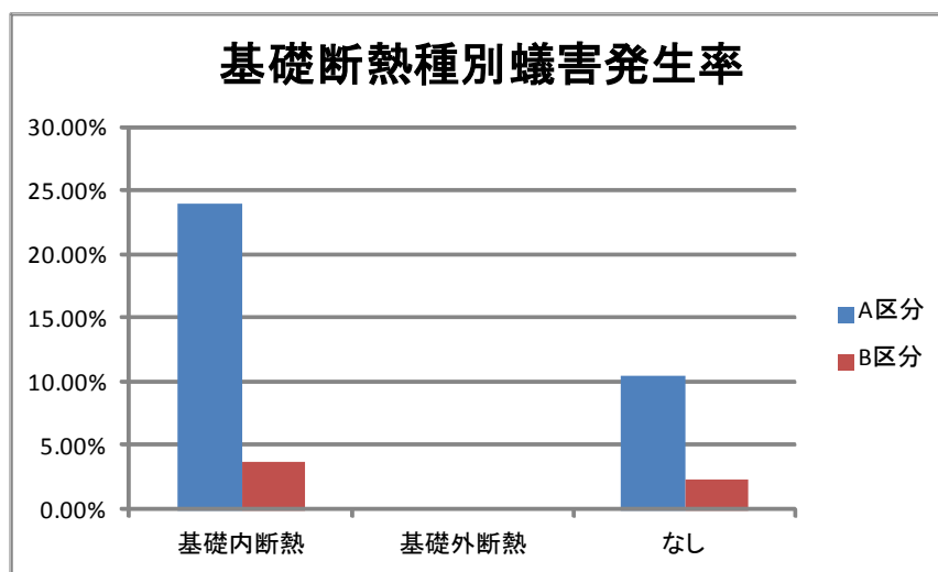
図 5-4 基礎断熱種別蟻害発生率
