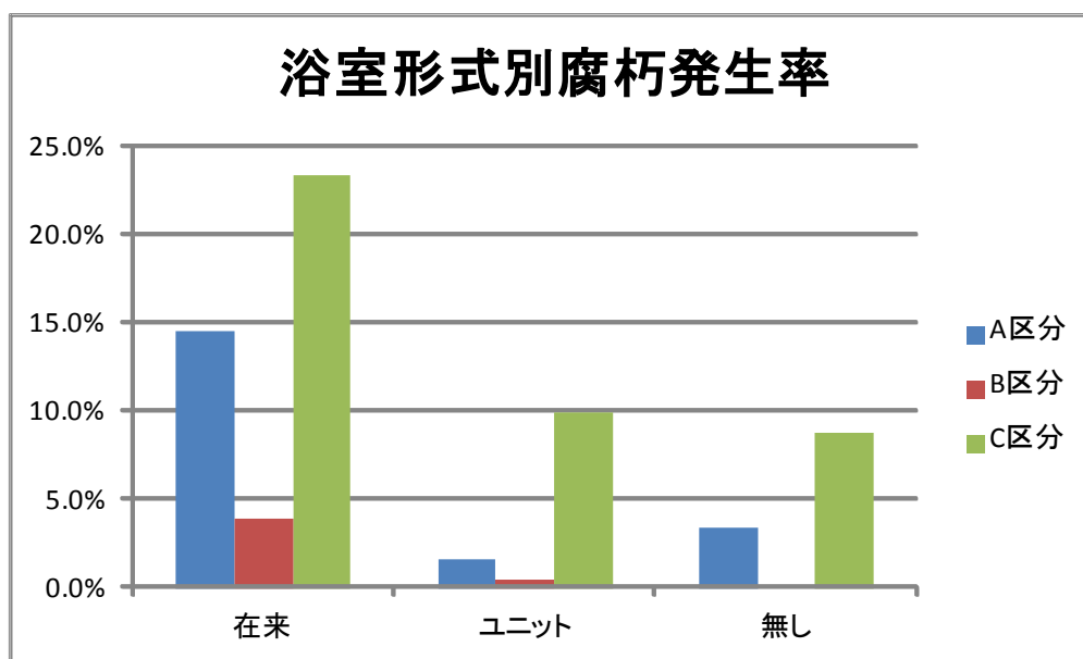
図 6-6 浴室形式別腐朽発生率
