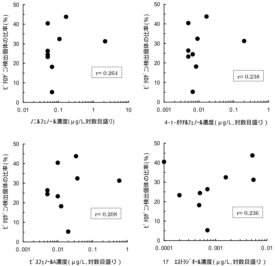
図 2.2.3 水質中の内分泌攪乱物質濃度とビテロゲニンが検出された雄コイの比率の関係（内分泌攪乱物質濃度は平成 10-13 年度調査結果の平均（検出下限未満の場合は検出下限の 1/2）、ビテロゲニンの検出比率は平成 10-13 年度調査全体の比率を用いた。図中の数値 (r) は相関係数を示す。）
