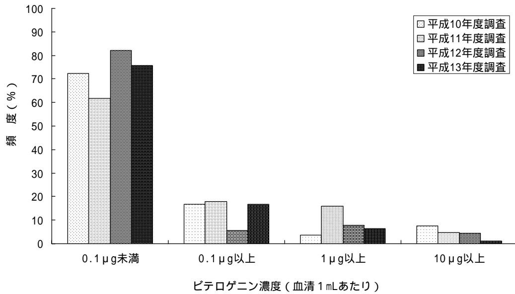
図 2.2.5 平成 10～13 年度調査での雄コイのビテロゲニン濃度 (平成 10～12 年度は、平成 13 年度と同じ 9 地点の結果を示した。)
