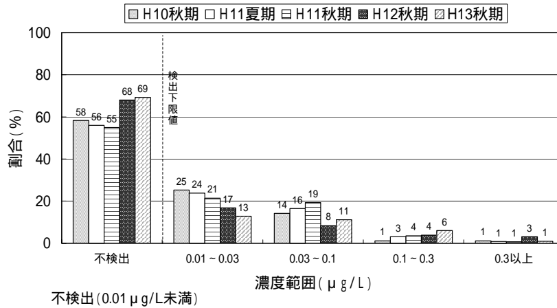
図 1.4.4 ビスフェノールAの濃度別分布
