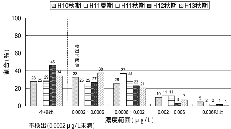
図 1.4.5 17-エストラジオール(ELISA法)の濃度別分布
