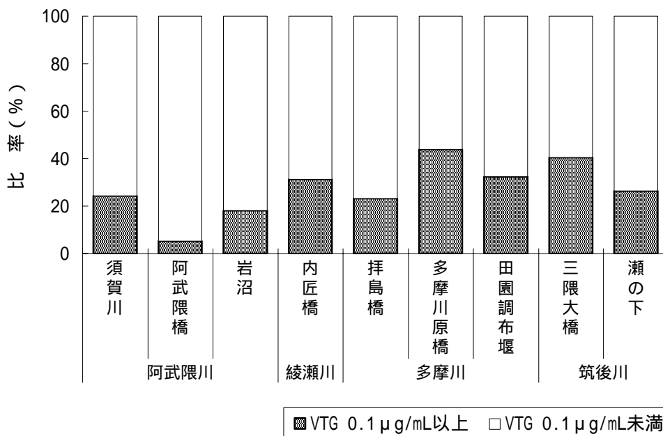
図 2.2.6 平成 10～13 年度調査全体での各調査地点の雄コイのビテロゲニン検出比率 (VTG 0.1 µg/mL 以上は、1 及び 10 µg/mL 以上もすべて含まれる)
