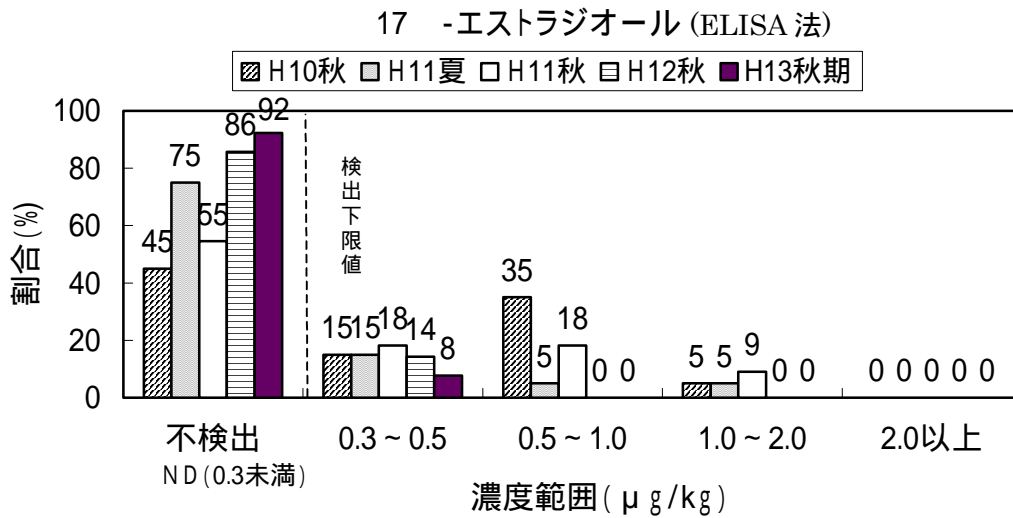
図 1.4.6 (2)濃度別頻度分布(底質・基本調査対象物質)
