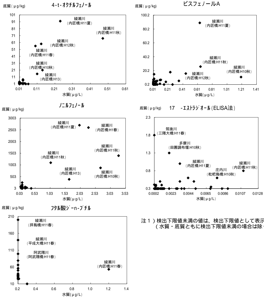
図 1.4.7 水質と底質の関係
