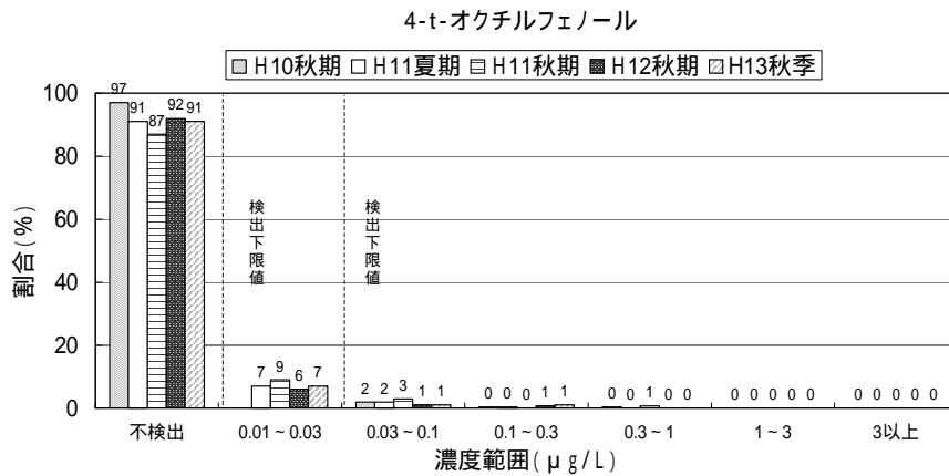
図 1.4.1 4-t-オクチルフェノールの濃度別分布
