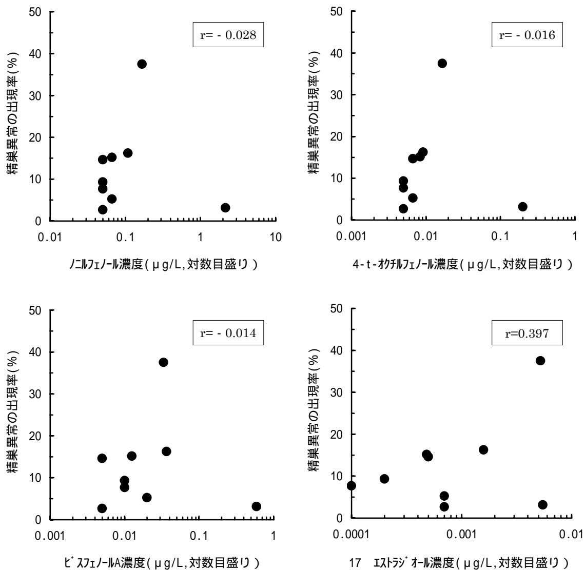
図 2.2.8 水質中の内分泌攪乱物質濃度と雄コイの精巢異常出現率の関係 (内分泌攪乱物質濃度は平成 10-13 年度調査結果の平均 (検出下限未満の場合は検出下限の 1/2) 精巢異常の出現率は平成 10-13 年度調査全体の比率を用いた。図中の数値(r)は相関係数を示す。)
