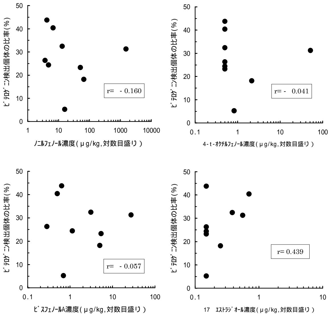
図 2.2.4 底質中の内分泌攪乱物質濃度とビテロゲンが検出された雄コイの比率の関係（内分泌攪乱物質濃度は平成 10-13 年度調査結果の平均（検出下限未満の場合は検出下限の 1/2）、ビテロゲンの検出比率は平成 10-13 年度調査全体の比率を用いた。図中の数値 (r) は相関係数を示す。）
