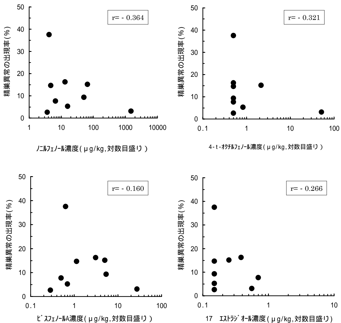
図 2.2.9 底質中の内分泌攪乱物質濃度と雄コイの精巢異常出現率の関係 (内分泌攪乱物質濃度は平成 10-13 年度調査結果の平均 (検出下限未満の場合は検出下限の 1/2)、精巢異常の出現率は平成 10-13 年度調査全体の比率を用いた。図中の数値( r )は相関係数を示す。)
