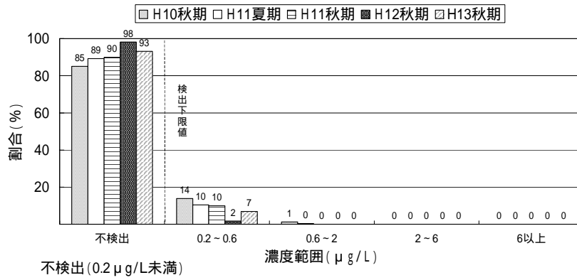
図 1.4.3 フタル酸ジ-n-ブチルの濃度別分布
