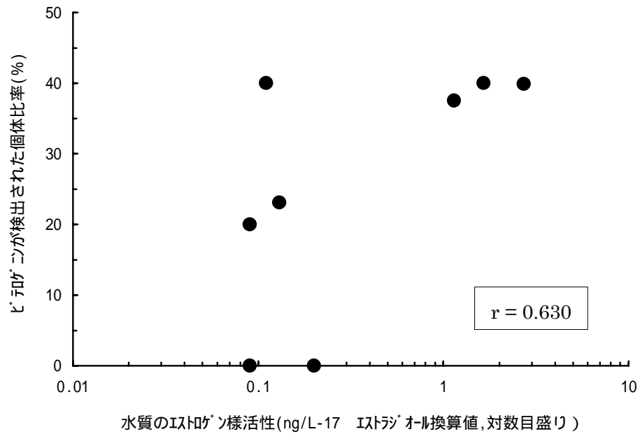
図 2.2.2(1) 水質中のエストロゲン活性様活性 (Sumpter 株での酵母法で測定) とビテロゲニンが検出された雄コイの比率の関係 (エストロゲン様活性及びビテロゲニンの検出比率は平成 13 年度調査の結果を用いた。図中の数値(r)は相関係数を示す。)
