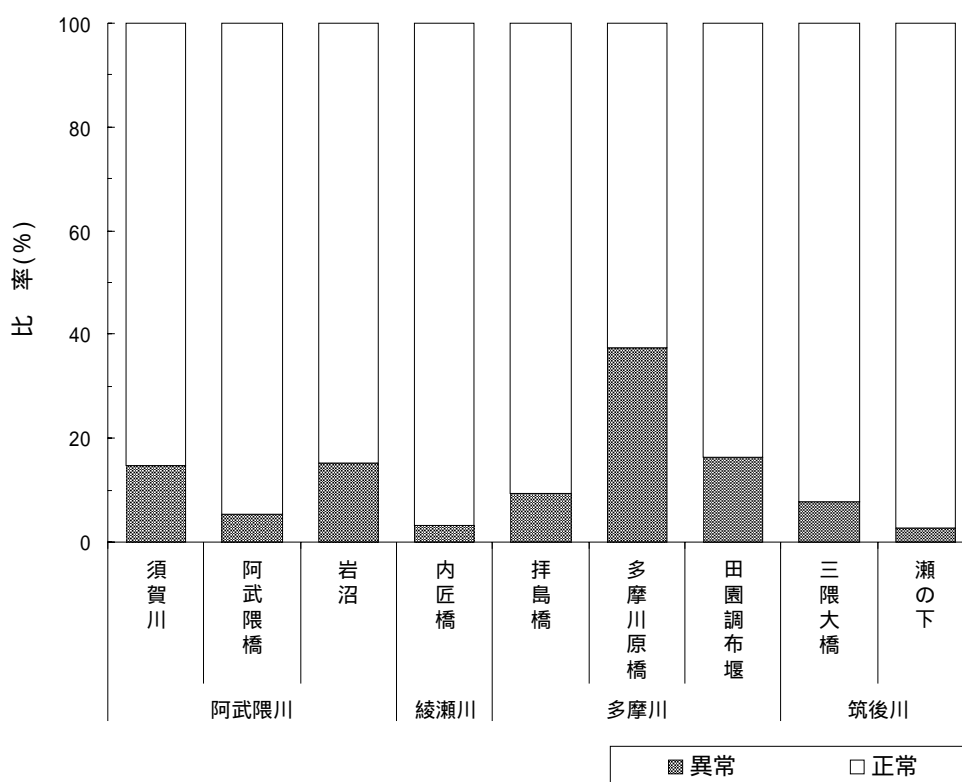
図 2.2.7 各調査地点の雄コイ精巢の観察結果 (平成 10～13 年度合計)
