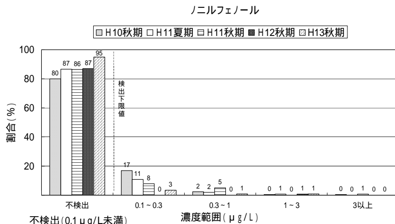
図 1.4.2 ノニルフェノールの濃度別分布
