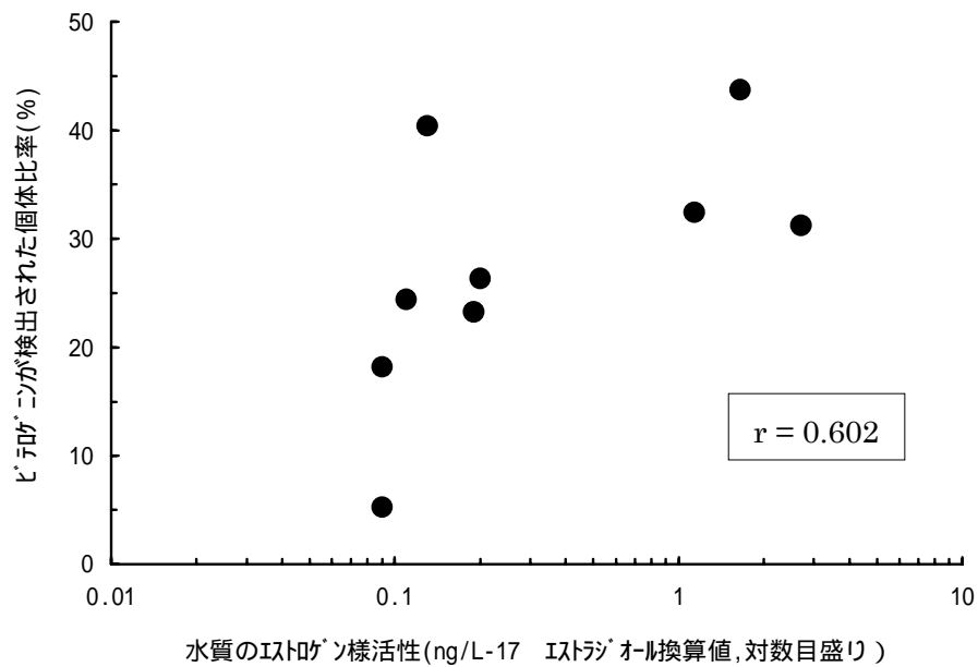
図 2.2.2(2) 水質中のエストロゲン活性様活性 (Sumpter 株での酵母法で測定) とビテロゲニンが検出された雄コイの比率の関係 (エストロゲン様活性は平成 13 年度調査、ビテロゲニンの検出比率は平成 10-13 年度調査全体の比率を用いた。図中の数値(r)は相関係数を示す。)
