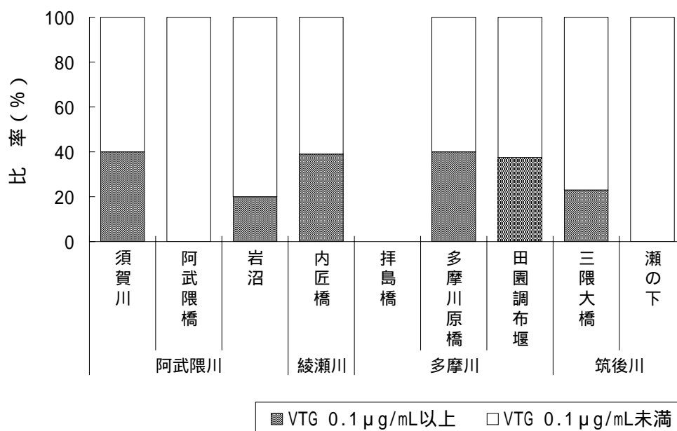
図 2.2.1 平成 13 年度調査での雄コイのビテロゲニン検出比率
