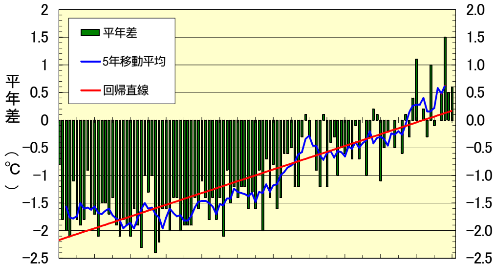
資料）気象庁福岡管区気象台 図 福岡の年平均気温平年差の経年変化
