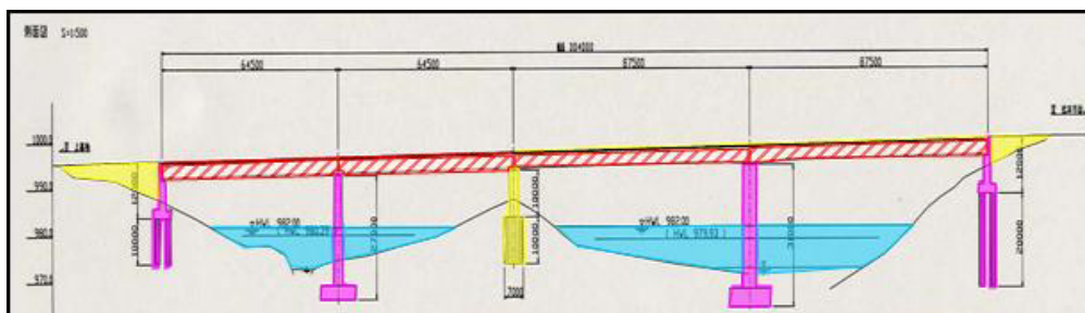
< 橋梁横断図 >
