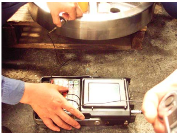
超音波探傷試験の実施状況(主ローラ) ※加工後に工場内で実施している状況
