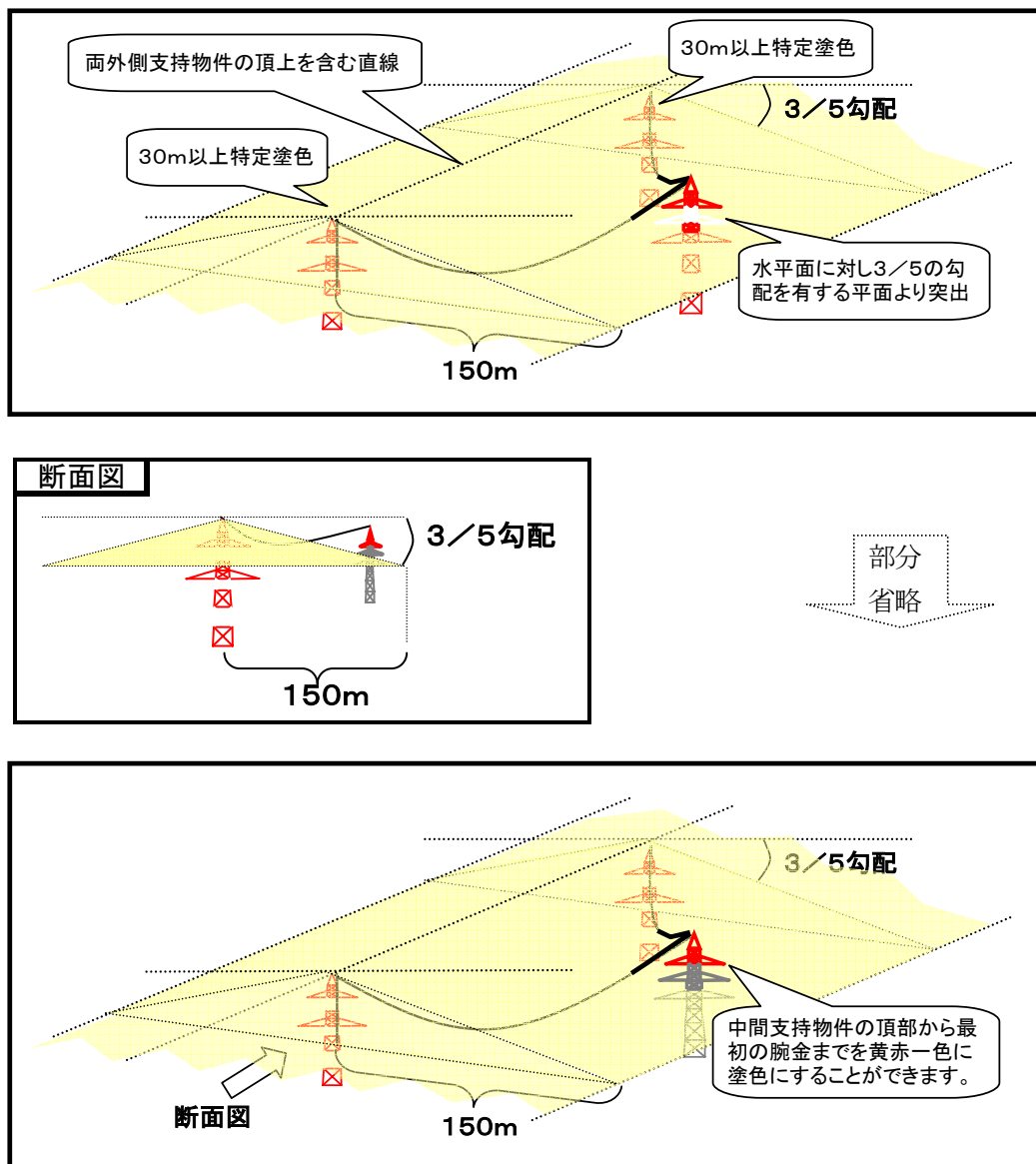
図5-26 2径間以上連続による部分省略(昼間障害標識)
