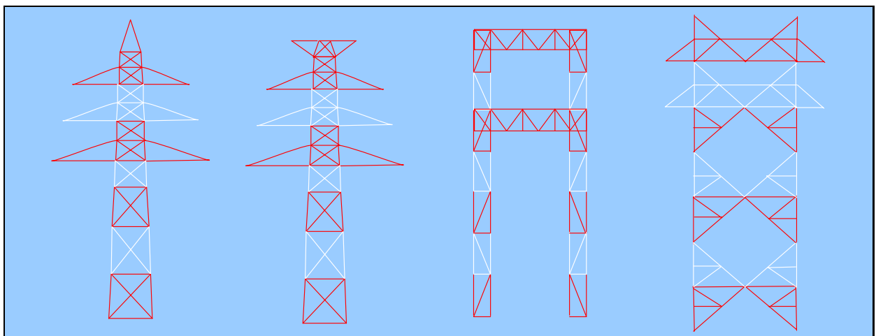
図6-25 球形標示物に代えて支持物件に塗色をする場合
