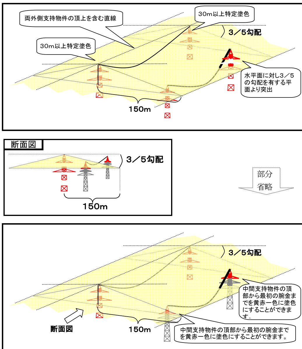
図5-27 近接による部分省略（昼間障害標識）
