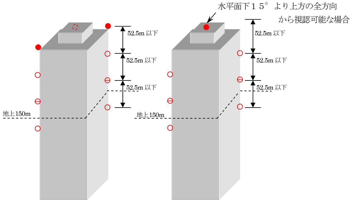
図6-8 塔屋類は3mを超え12m以下の物件
