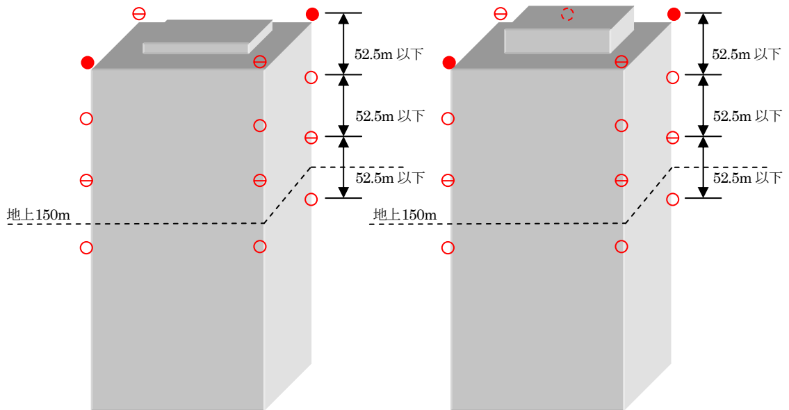
図6-9 塔屋類は3m以下の物件
