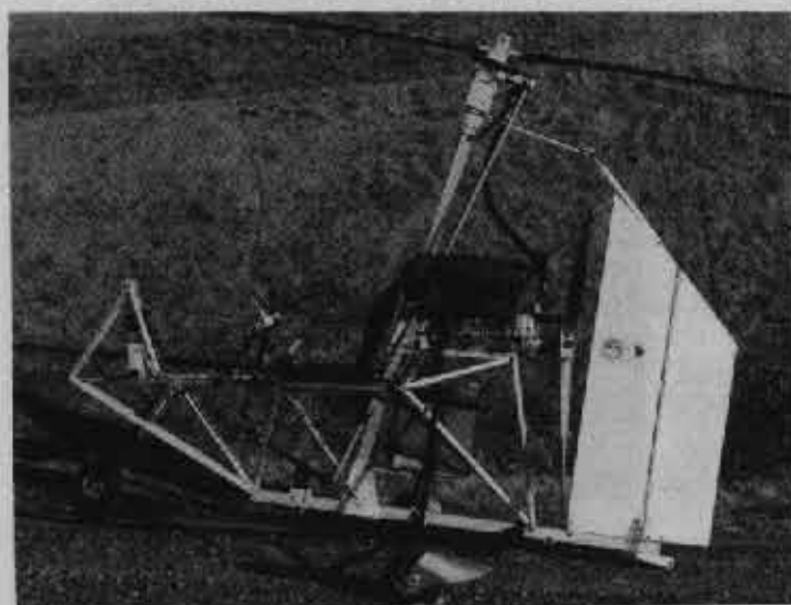
側面写真 (基本仕様)
