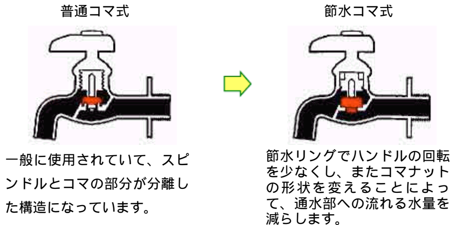
図 節水コマの仕組み
