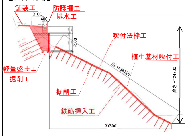
【断面図】 A-A' 断面
