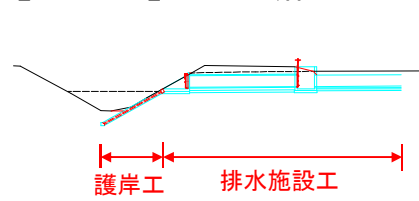
【断面図】 A-A' 断面
