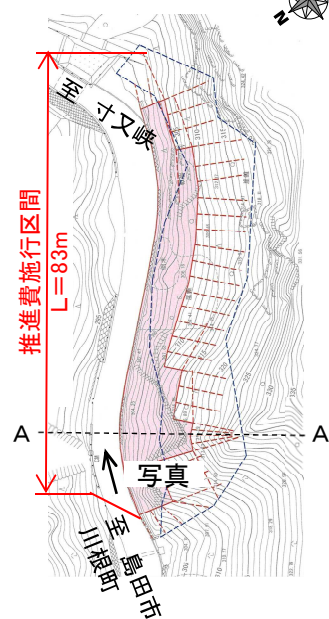
【平面図】
