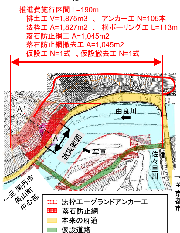
【平面図】
