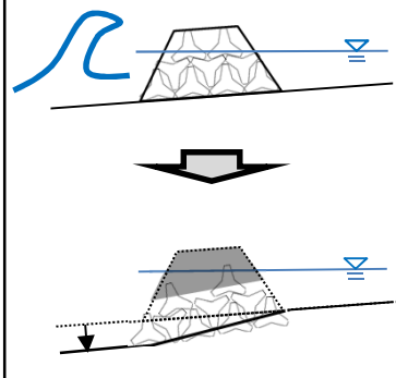
【波浪による沈下イメージ図】
