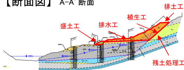
【断面図】 A-A' 断面
