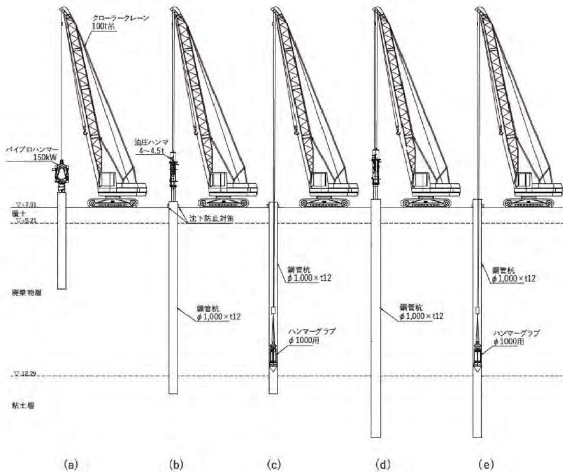
図-8 Case3の施工イメージ
