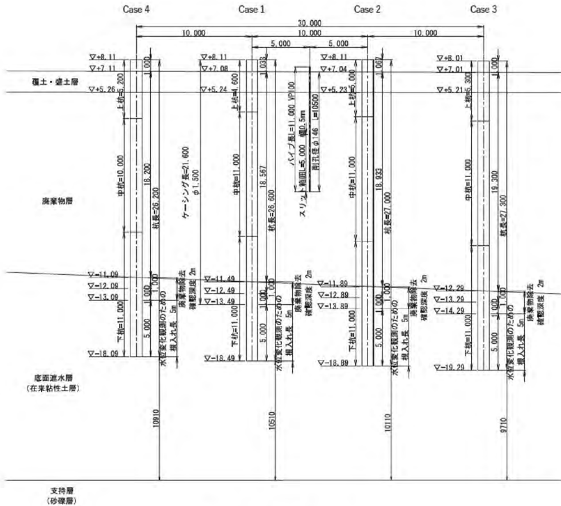
図-5 試験杭の施工計画図
