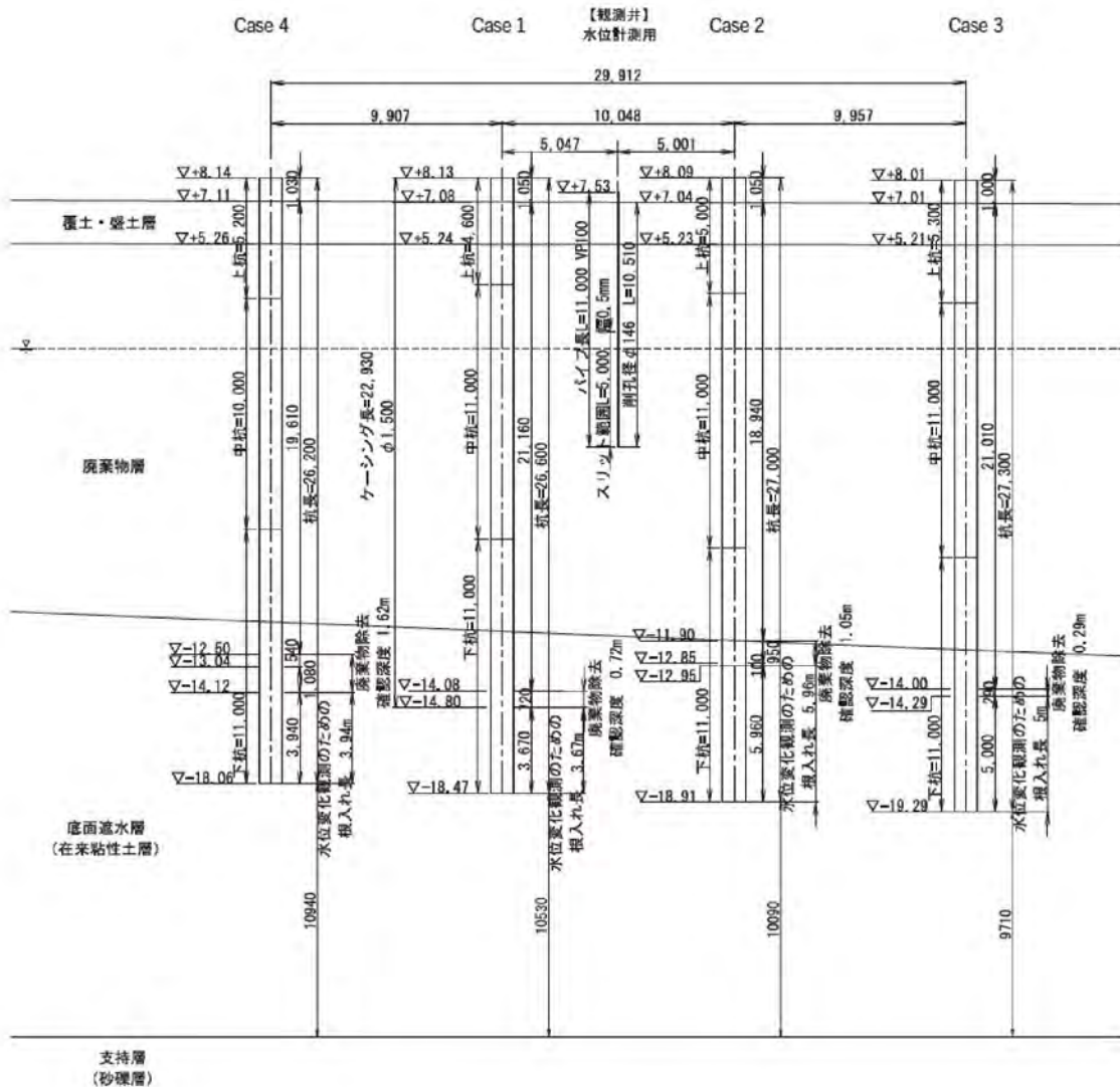
図-10 施工出来形図
