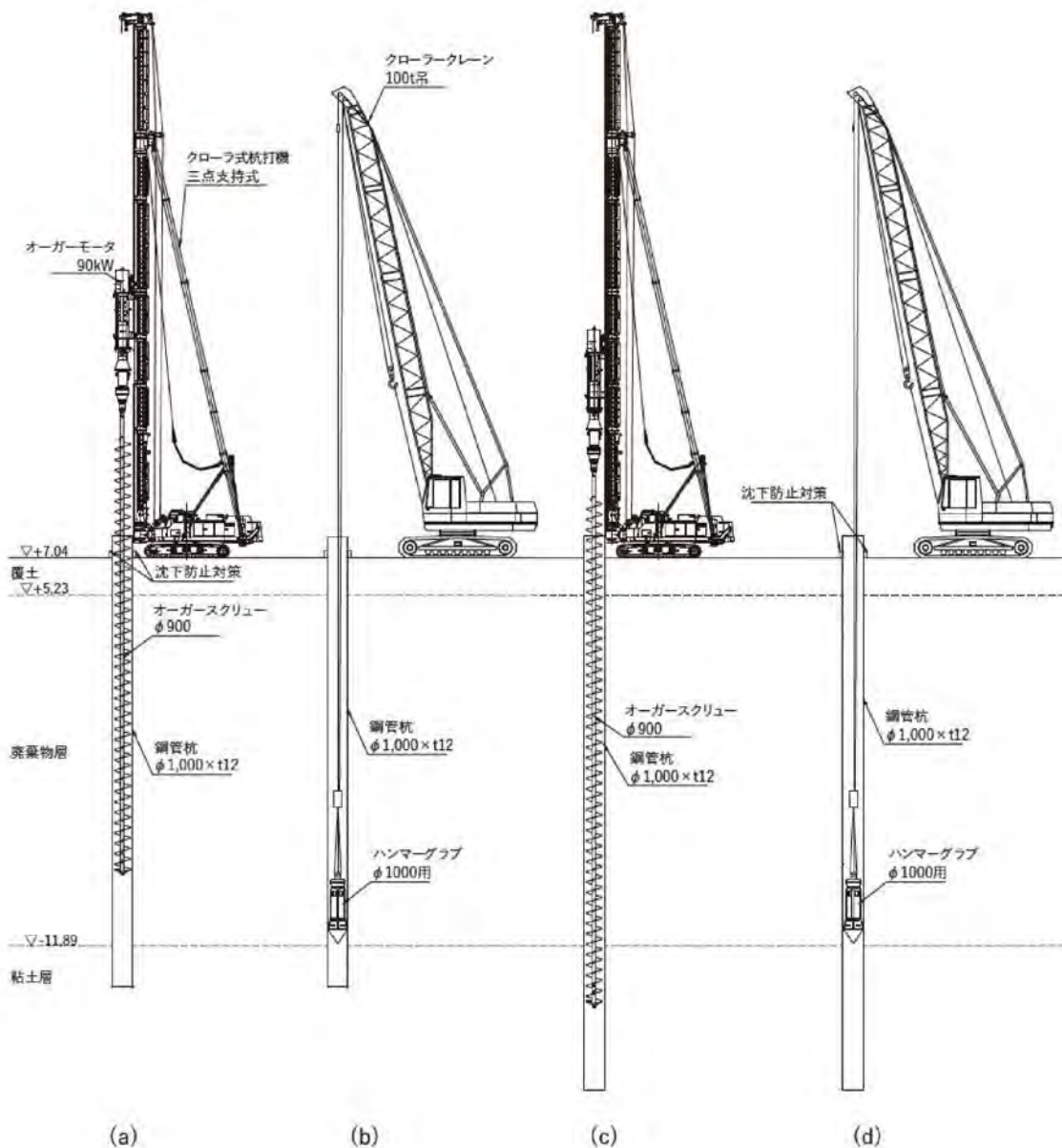
図-7 Case2の施工イメージ
