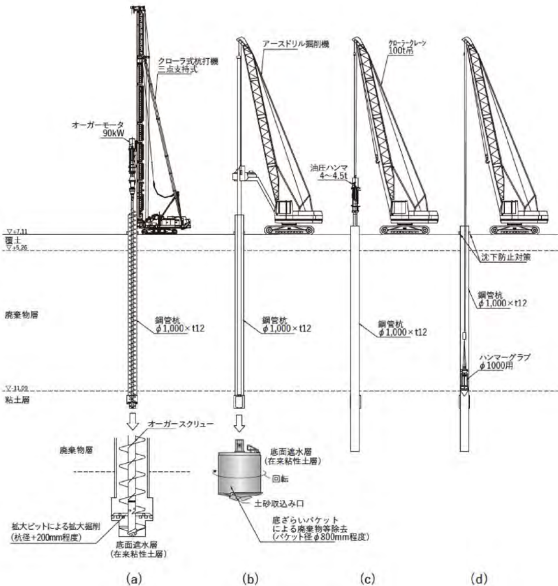
図-9 Case4 の施工イメージ
