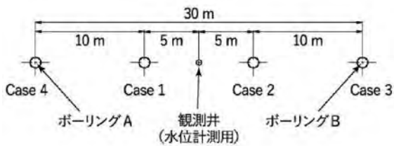
図-2 ボーリング実施位置
