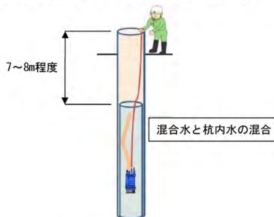
図 2-4 混合水と杭内水の混合
