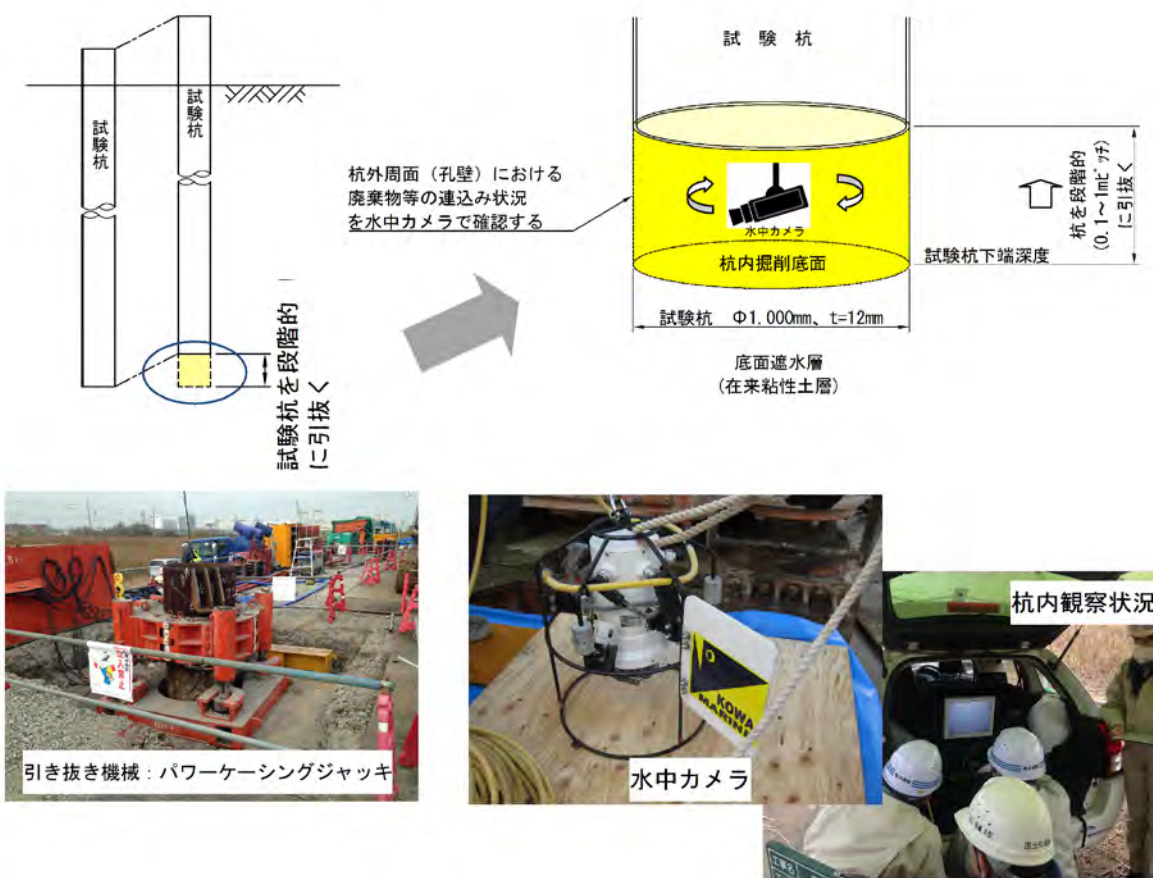
図 1-2 試験杭引抜き時の観察実施イメージ図
