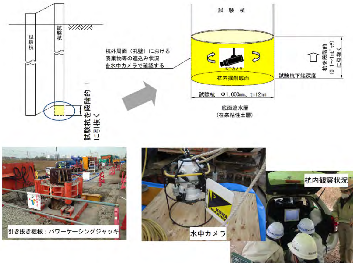
図 2-1 試験杭引抜き時の観察実施イメージ図
