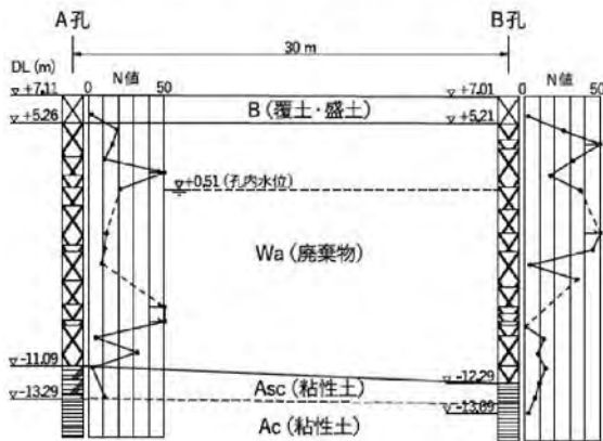
図-3 土層縦断面図
