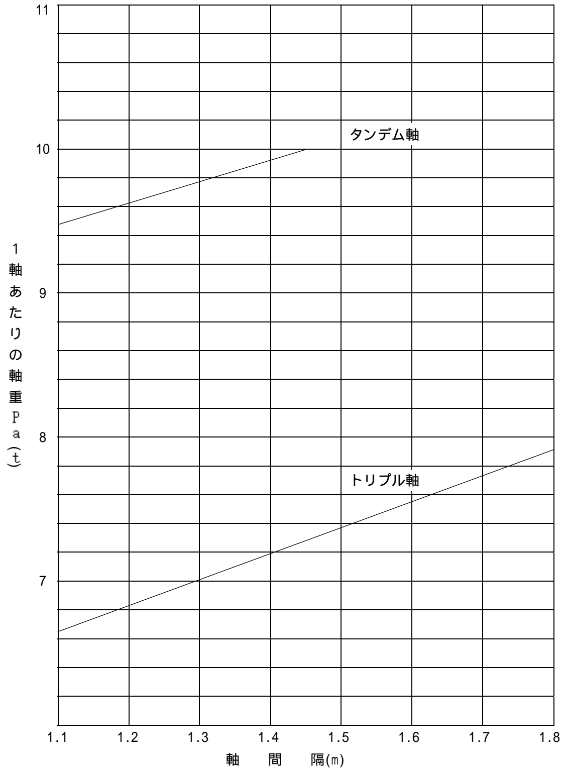
図2 設計荷重がTL 20設計荷重以上である道路
