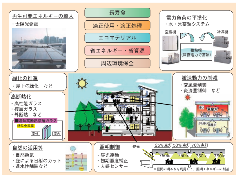
図表Ⅱ-7-1-6 環境に配慮した庁舎のイメージ図
