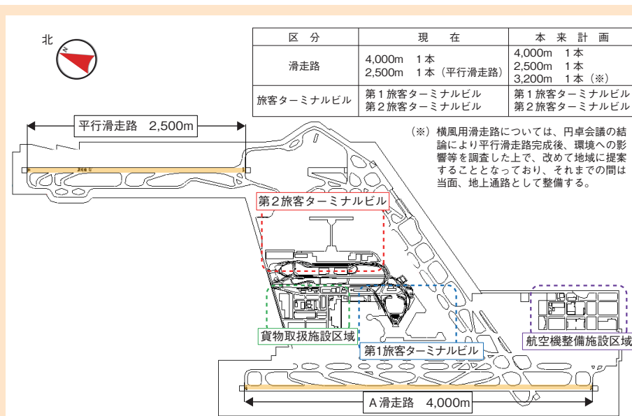
図表Ⅱ-5-1-9 成田国際空港の施設計画
