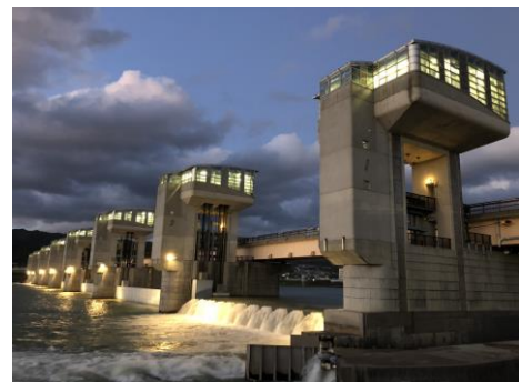
紀の川大堰（和歌山県）
