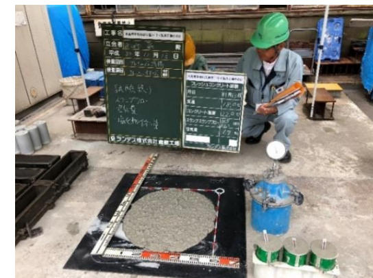
フレッシュ性状試験状況
