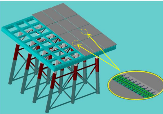
工法概要図
