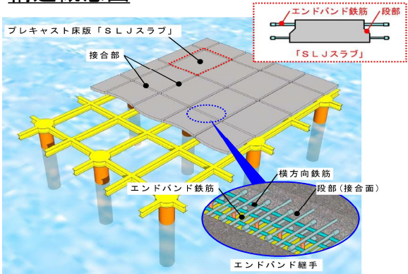
横方向鉄筋の仮配置
