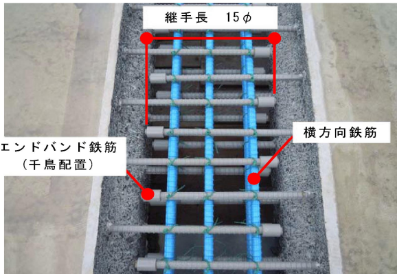
場所打ち部配筋状況
