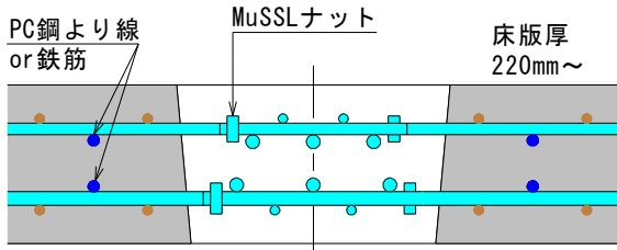
継手部断面図
