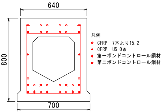
PCホロー桁断面図(例)
