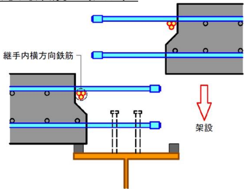
場所打ち部配筋状況
