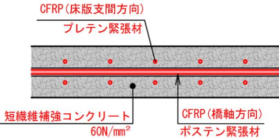
CFRPスラブ 断面構成図
