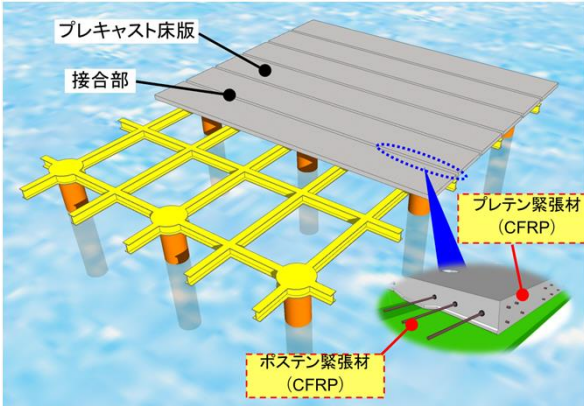
実績事例: 許田高架橋他1橋床版取替工事(その2). (注)道路橋床版での適用事例
