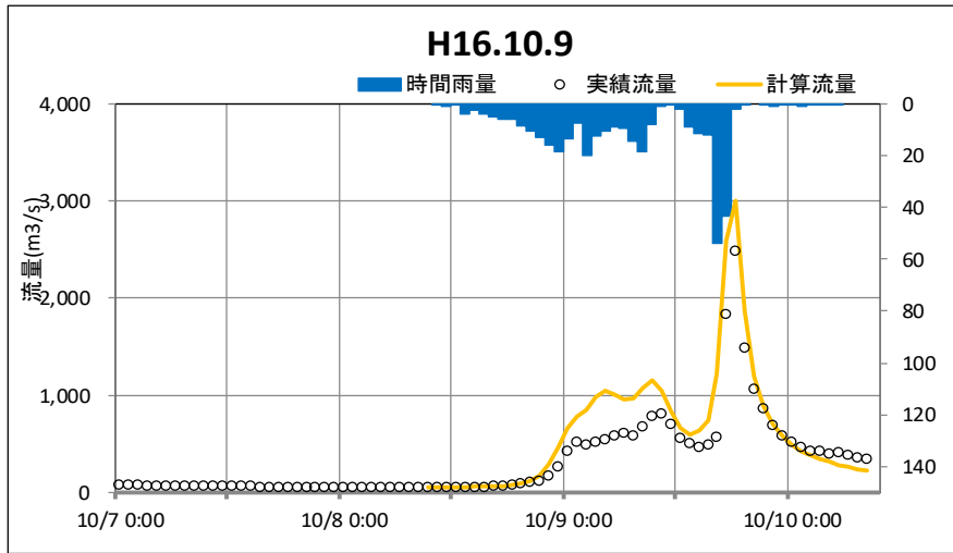
図 1-8-5 平成 16 年 10 月洪水再現計算結果
