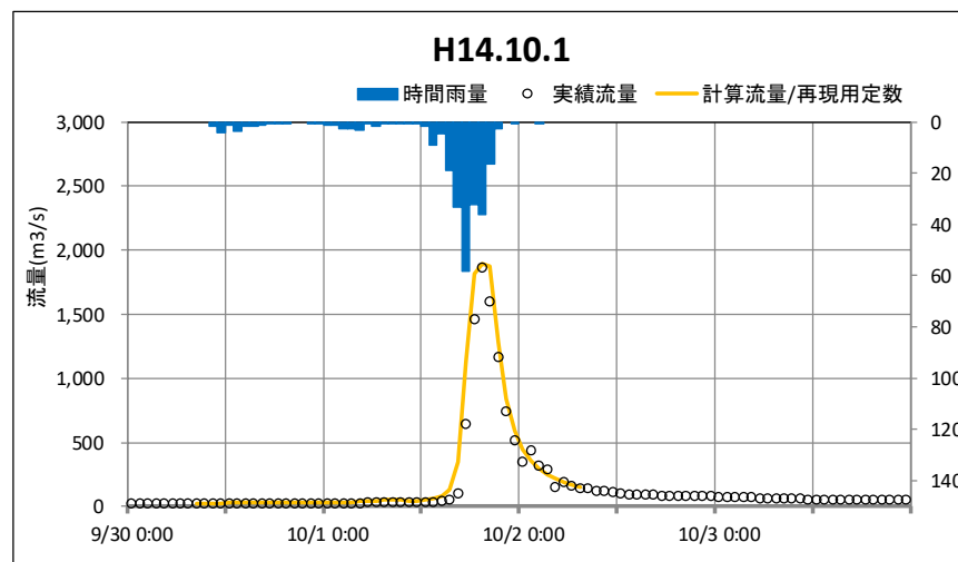
図 1-8-4 平成 14 年 10 月洪水再現計算結果
