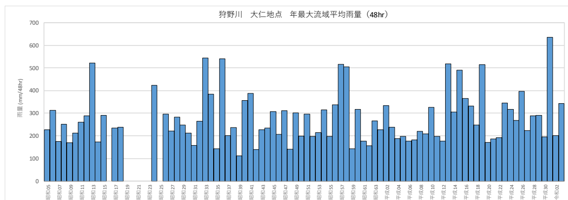
図 1-4-2 年最大流域平均雨量 (基準地点大仁上流域)
