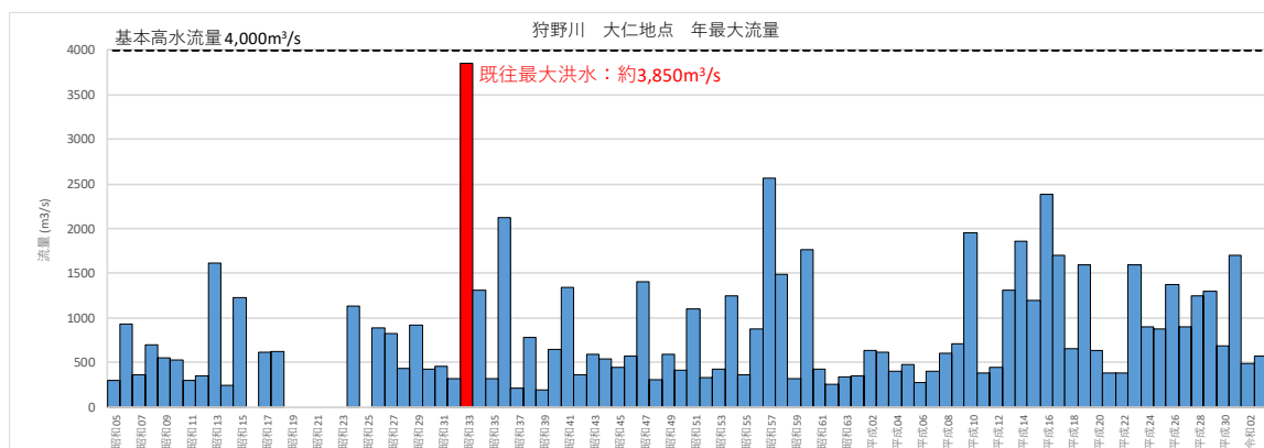
図 1-4-1 年最大流量 (基準地点大仁)
