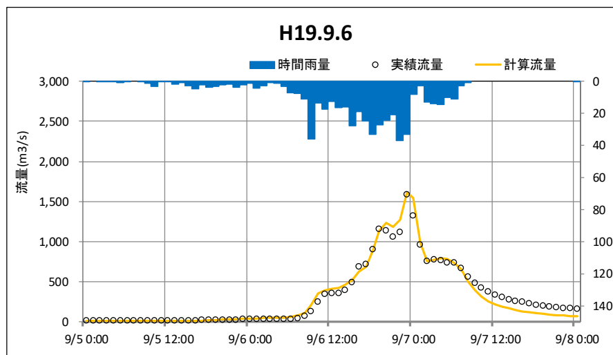
図 1-8-7 平成 19 年 9 月洪水再現計算結果
