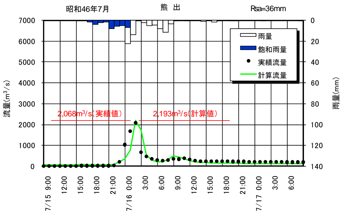
図 4-9 昭和 46 年 7 月洪水再現計算結果（熊出地点）
