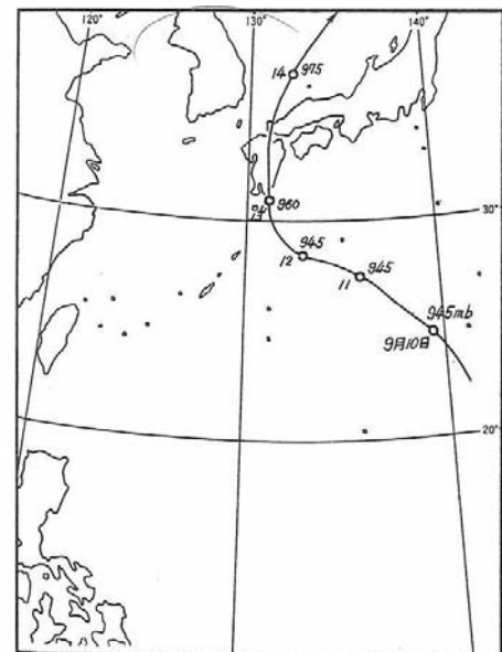
図4-2 台風経路図（昭和25年9月洪水）
