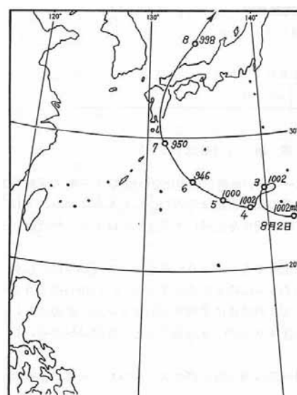
図4-3 台風経路図（昭和29年9月洪水）
