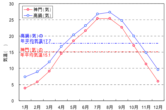
図 1-7 代表地点の月別平均温度(1997～2006年の平均)
