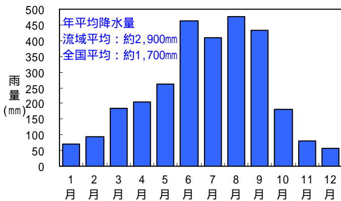
図 1-4 月別平均降水量 (1985～2006年の平均)
