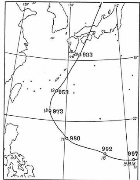
図4-1 台風経路図（昭和18年9月洪水）
