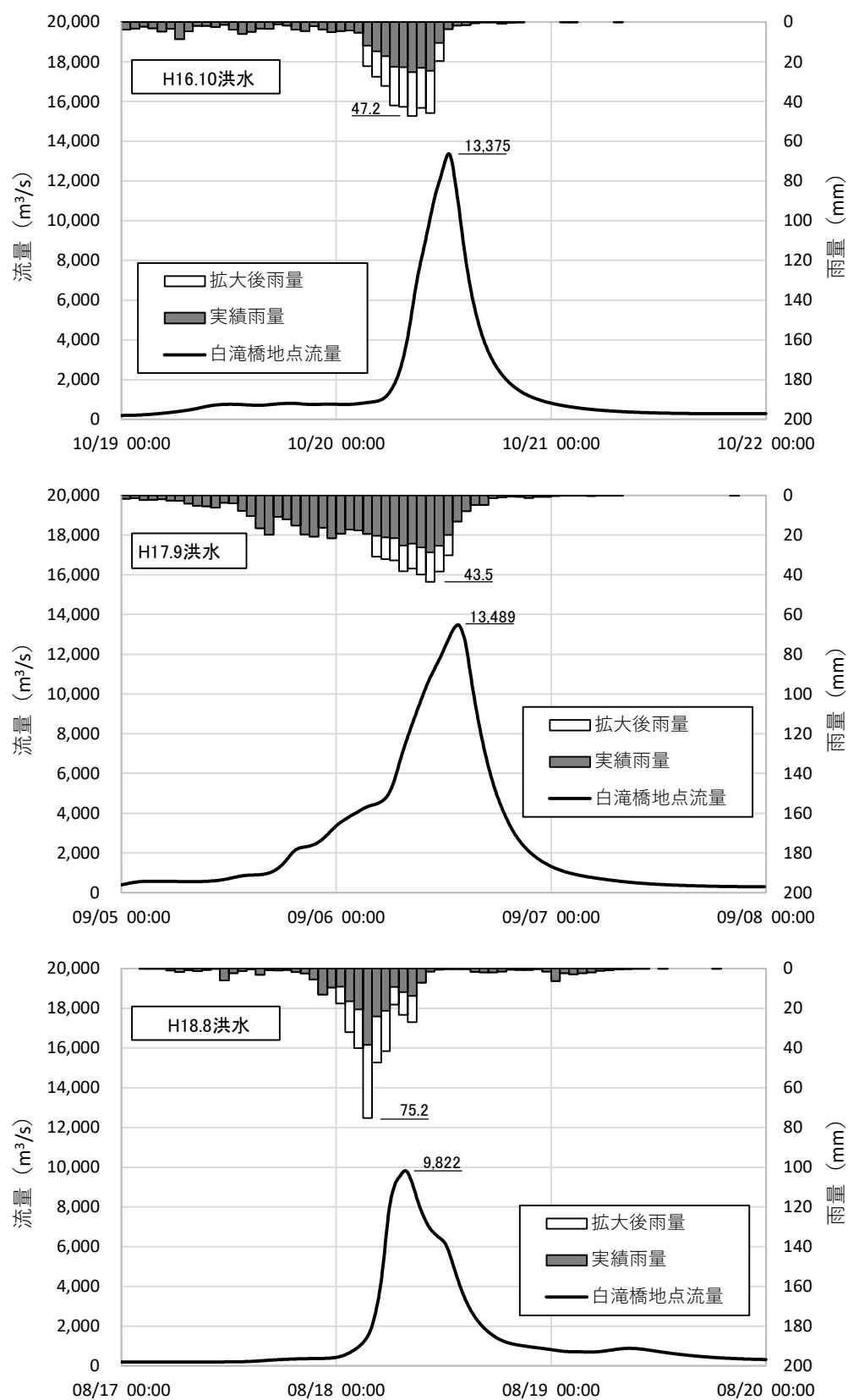
図 1.23 (4) 基本高水ハイドログラフ
