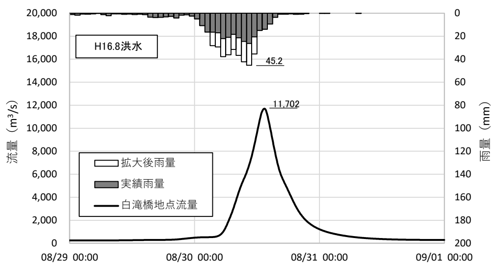
図 1.23 (3) 基本高水ハイドログラフ
