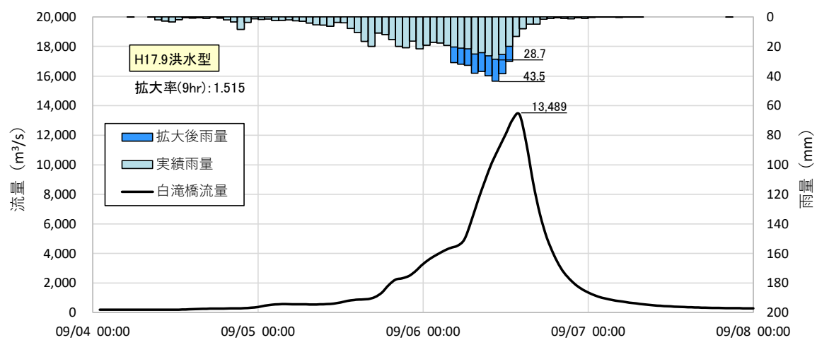
図 1.31 基本高水（平成 17 年 9 月洪水：白滝橋）
