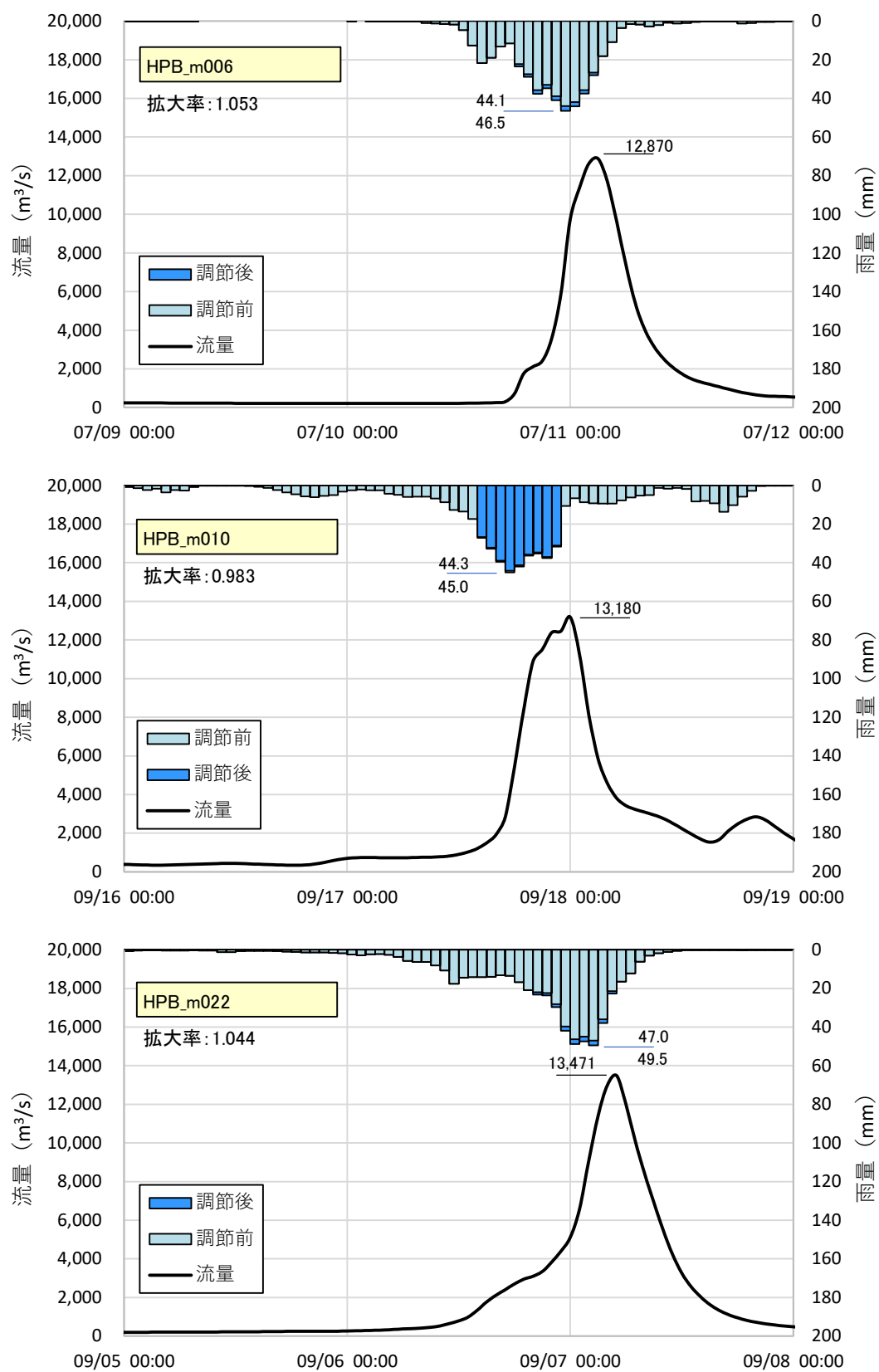
図 1.25 (4) アンサンブル予測降雨波形における流出計算結果
