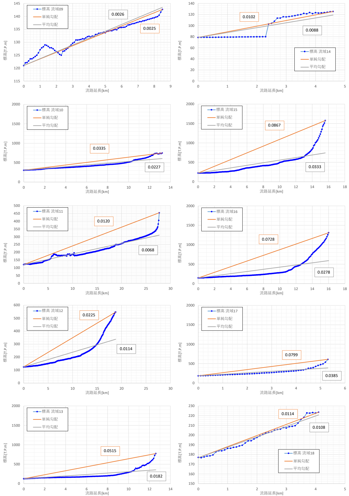
図 1.13 (2) 流域平均勾配の算定結果
