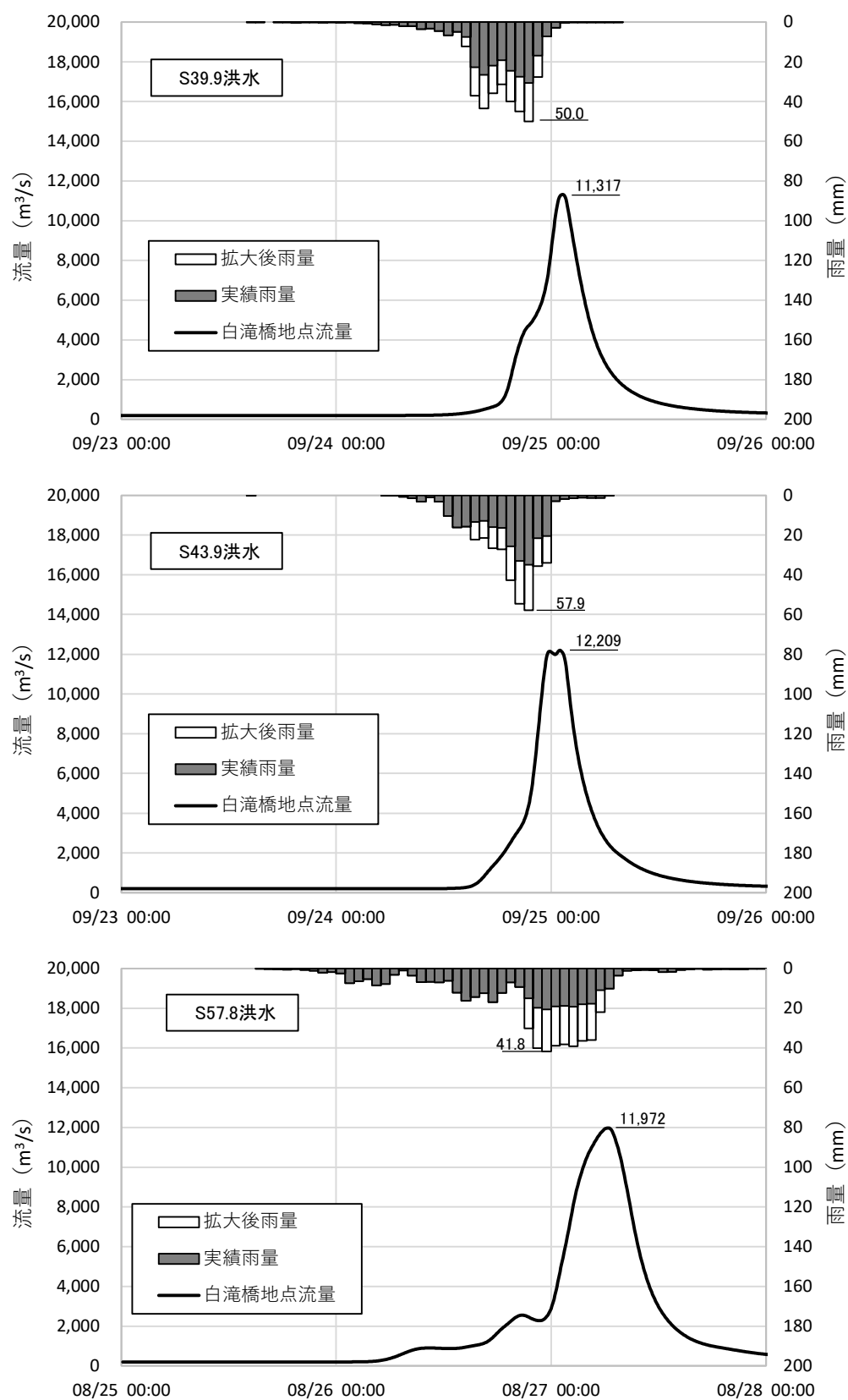
図 1.23 (2) 基本高水ハイドログラフ
