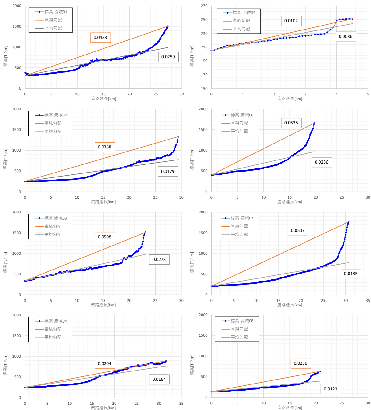
図 1.13 (1) 流域平均勾配の算定結果
