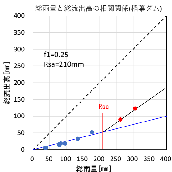
図 1.8 総降雨量と総流出高の関係
