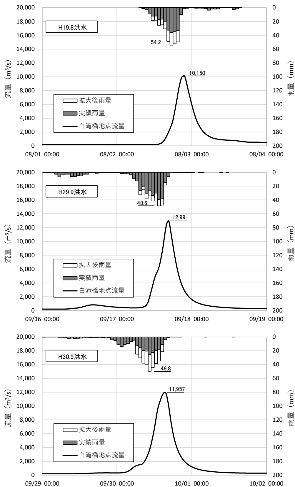
図 1.23 (5) 基本高水ハイドログラフ
