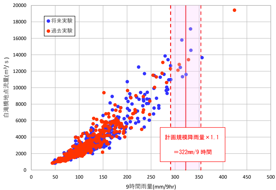
図 1.24 アンサンブル予測降雨波形からの抽出（基準地点白滝橋）
