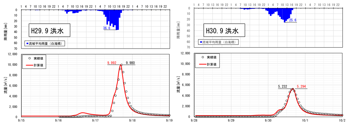
図 1.14 (3) 再現計算結果 (白滝橋)
