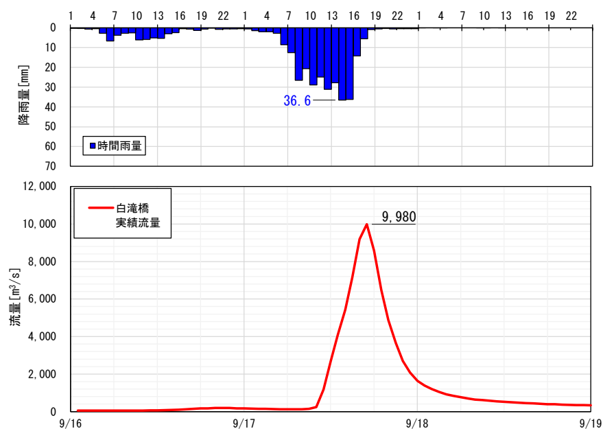
図 1.29 平成 29 年 9 月洪水（基準地点白滝橋）
