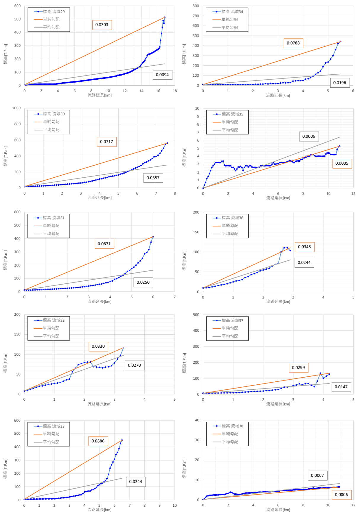
図 1.13 (4) 流域平均勾配の算定結果
