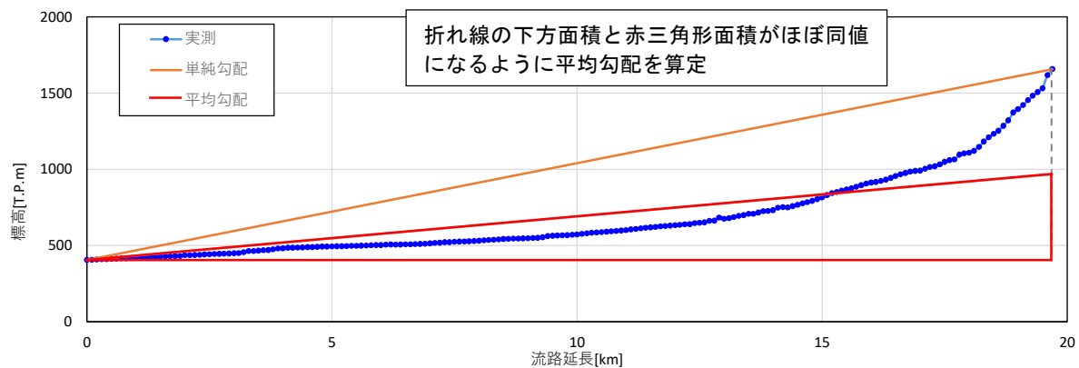
図 1.12 流域平均勾配の設定例
