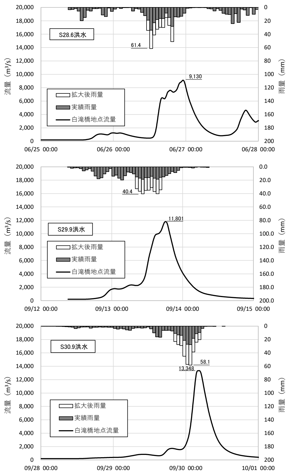
図 1.23 (1) 基本高水ハイドログラフ
