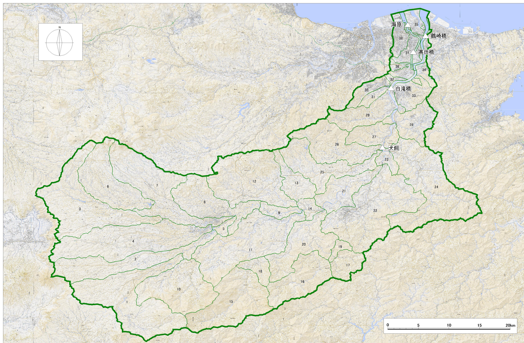
图 1.3 流域分割图
