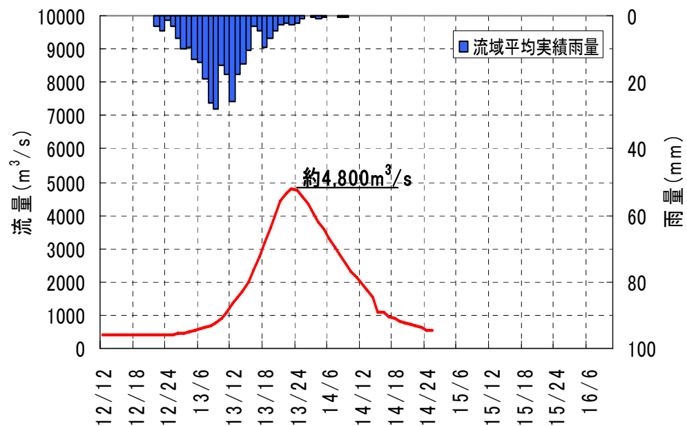
図 4-15 平成 7 年 7 月洪水流域湿潤状態での平成 16 年 7 月洪水の検証（下流部）
