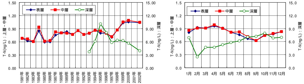
図 6.2.9 小川原湖における層別年平均値・月平均値の推移状況(T-N)
