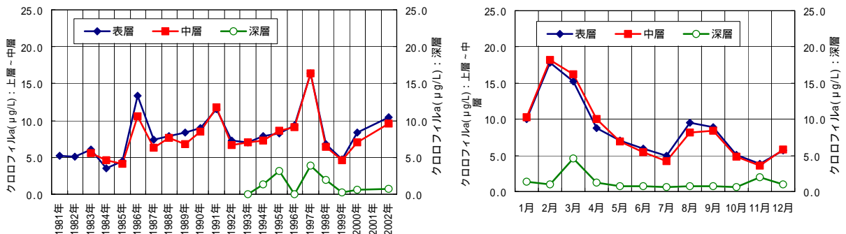
図 6.2.8 小川原湖における層別年平均値・月平均値の推移状況(クロロフィル a)
