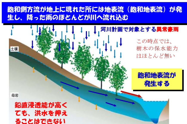
図-3 大雨時の森林斜面からの流出量 (東京大学名誉教授・福島大学教授 虫明功臣「森林斜面から溪流や河川への流出過程」より)
