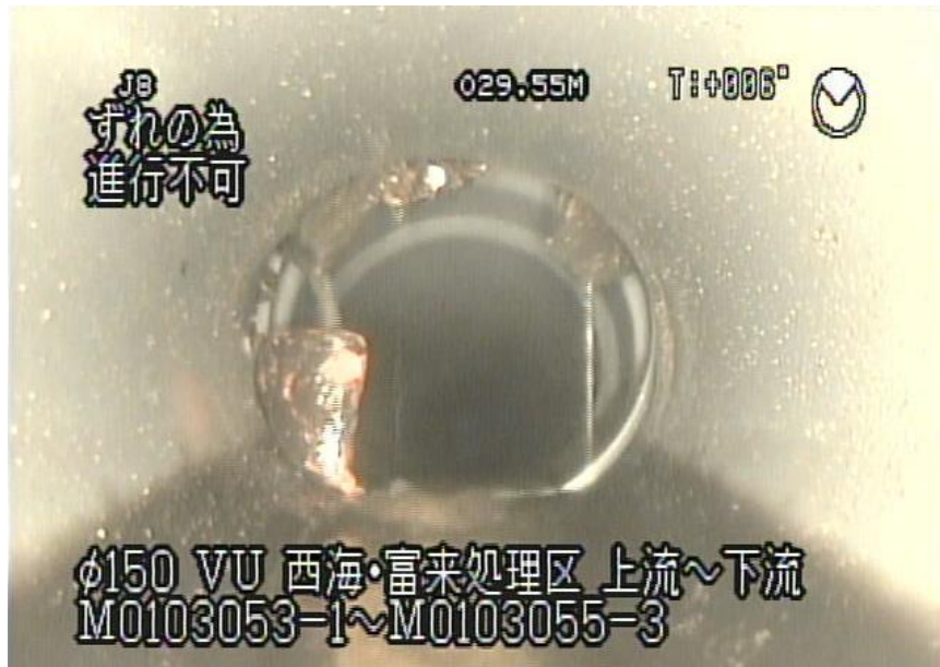
■ 2/3 2次調査(TVカメラ調査における管内の様子)(志賀町)
