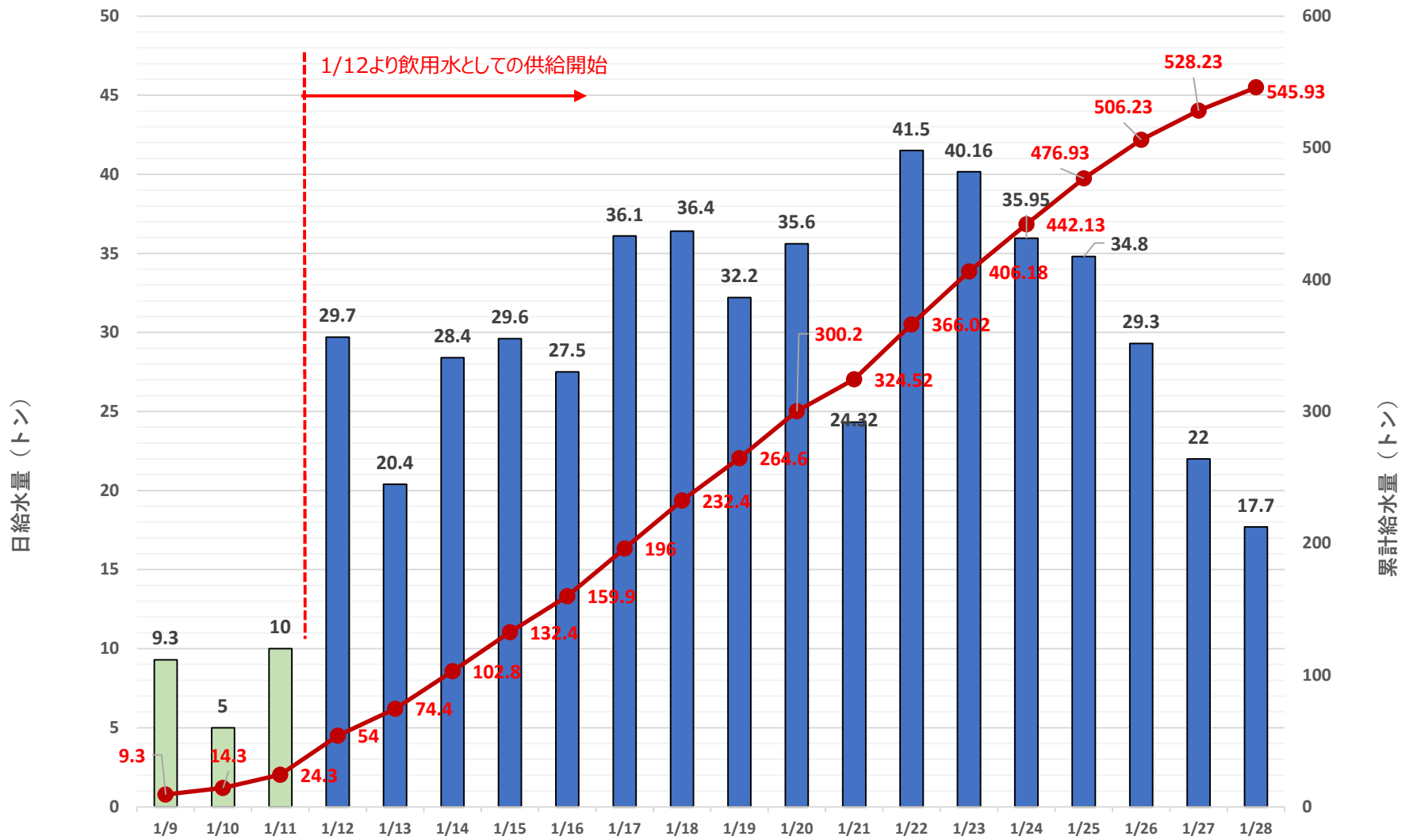
令和6年能登半島地震 可搬式浄水装置による給水支援
