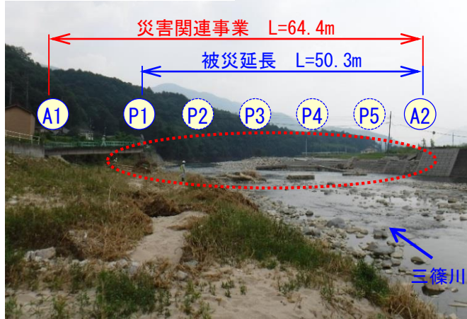
全景（5径間落橋/6径間）
