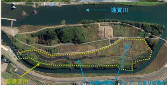
上. 河川の縦断的連続性の保全・再生 遠賀川河口堰の多自然魚道 中. 河川とその周辺の横断的連続性の再生 御徳地区における樋管の落差解消 下. 河川における湿地環境の再生 中島地区の自然再生事業 左. 遠賀川流域に飛来したコウノトリ(令和4年11月撮影)
