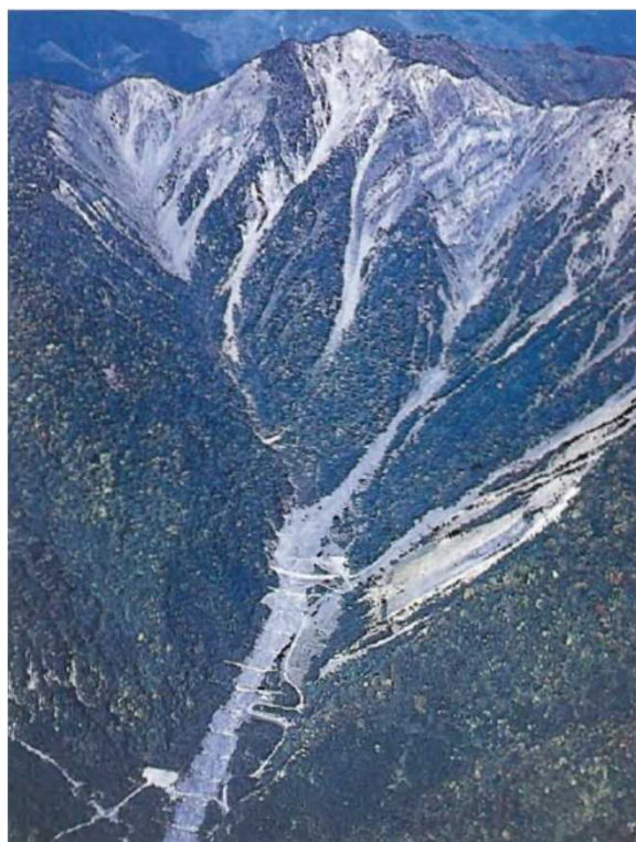
●安倍川上流の大谷崩れと床固工群（静岡県静岡市）
