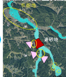
施設配置計画の見直し
