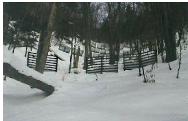
● 雪崩予防柵工(長野県松本市安曇)
