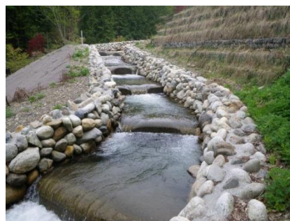
●魚類に配慮した金原砂防堰堤に設置された魚道とその観察窓（長野県）
