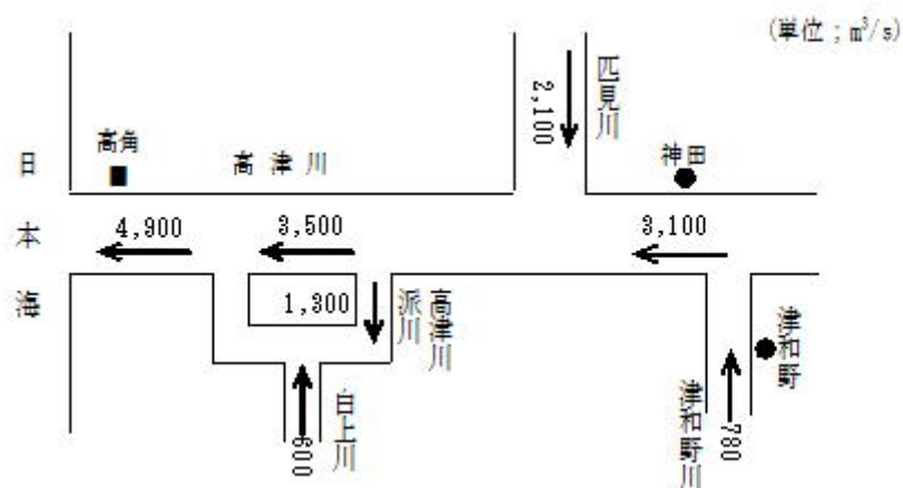
高津川計画高水流量図
