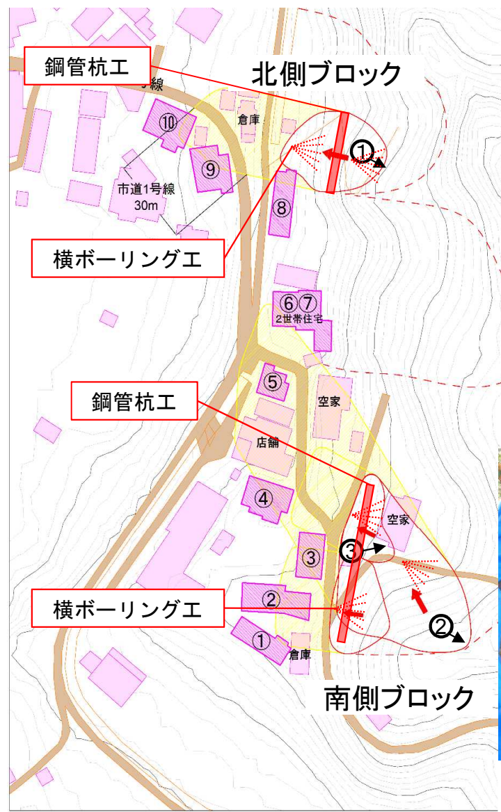
平面図(対策イメージ)
