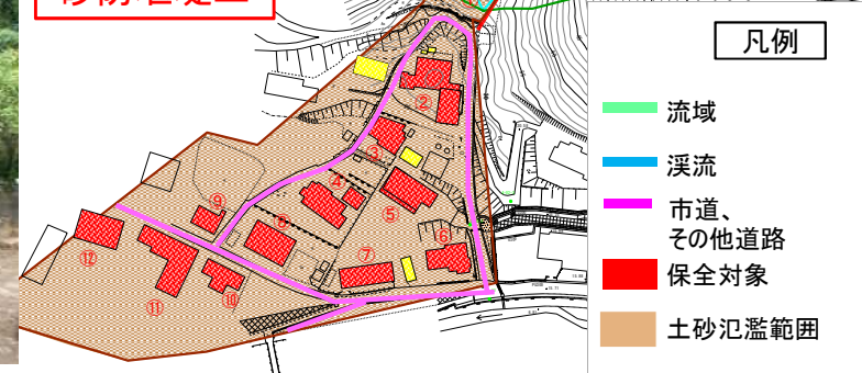
砂防堰堤工
