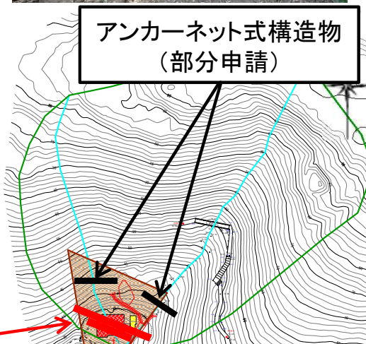
砂防堰堤工
