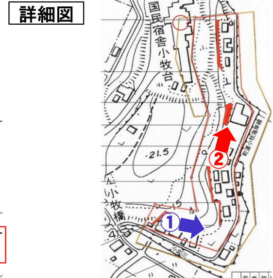
②対策済み斜面 (S57~60年度施工)【R6.1.9撮影】 (擁壁工を施工した人家裏の斜面では崩壊を防止) 《対策済み箇所》
