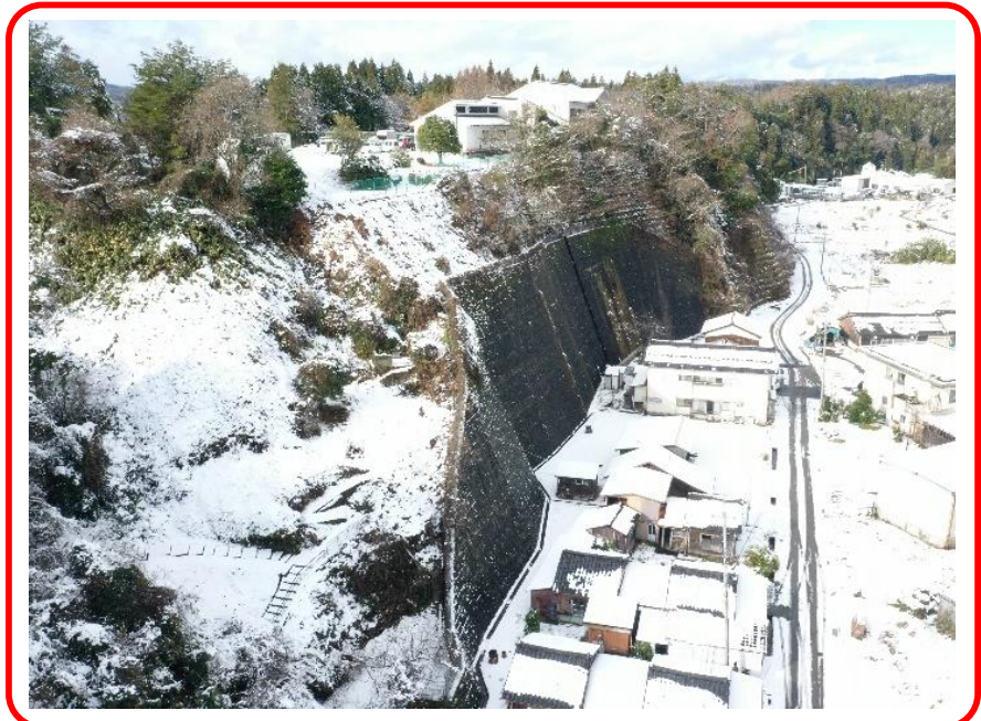
②対策済み斜面 (H5~9年度施工)【R6.1.6撮影】 (擁壁工を施工した人家裏の斜面では崩壊を防止) 《対策済み箇所》
