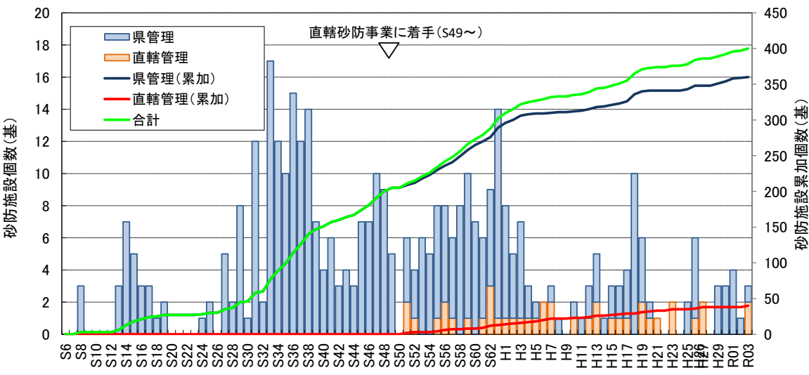
日野川流域内の砂防堰堤数の経年変化
