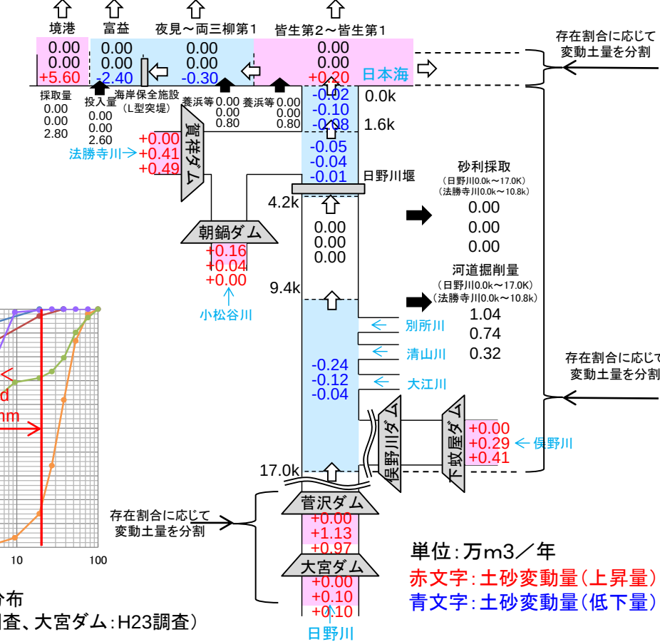
土砂動態②:平成～令和年代【粒径考慮】 (ダム6施設、河道樹林化後・日野川堰改築後、海岸保全施設あり)
