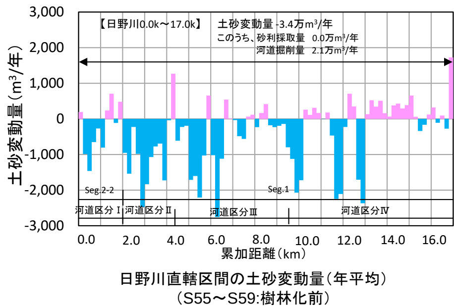
土砂動態①: 昭和年代～平成初期(河道樹林化前)
