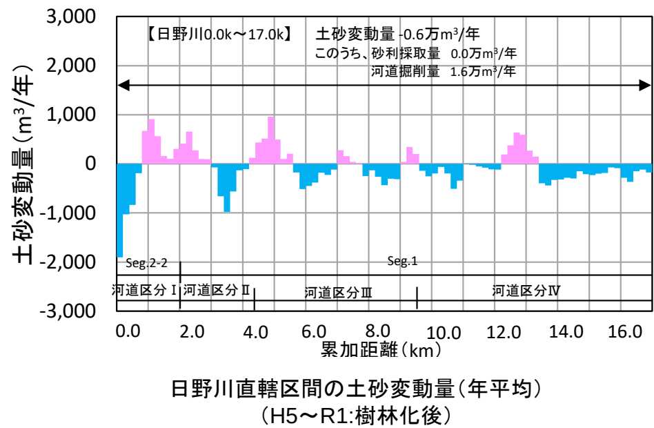
土砂動態②: 平成初期～令和年代(河道樹林化後)
