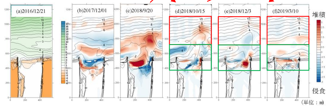
図・6 侵食堆積図 (2016/12/21~2019/3/10)
