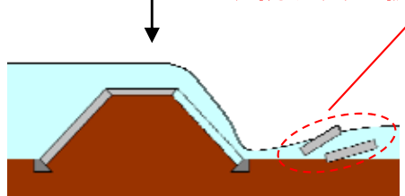
堤防裏法の被覆工の流出
