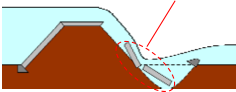
裏法部の被覆工の流出
