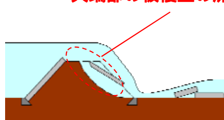
天端部の被覆工の流出
