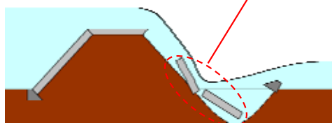
裏法部の被覆工の流出
