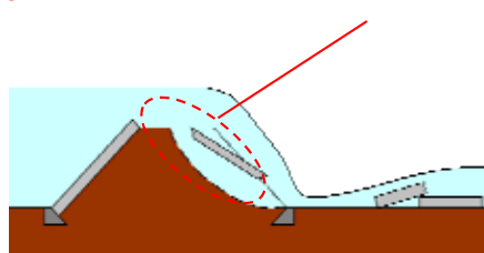
天端部の被覆工が流出
