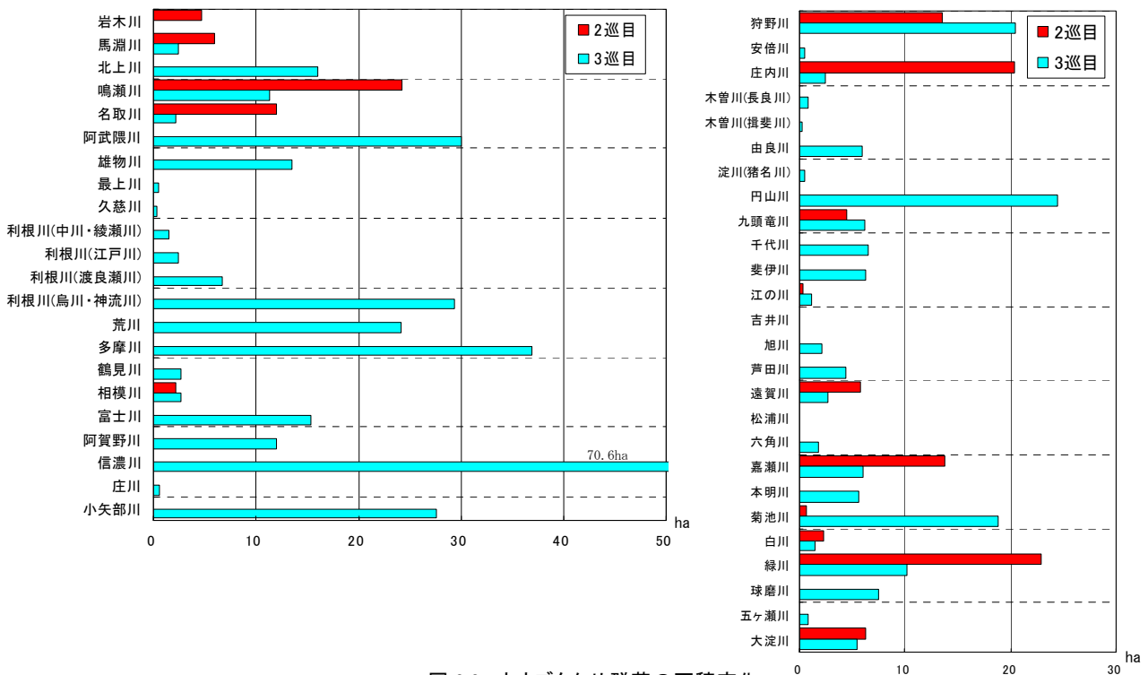
図 3.3 オオブタクサ群落の面積変化
