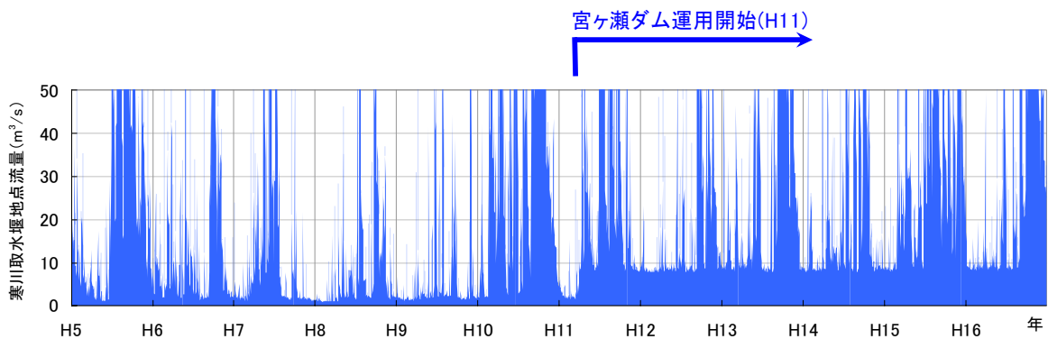
図 3.15 相模川におけるダム運用による流況改善効果
