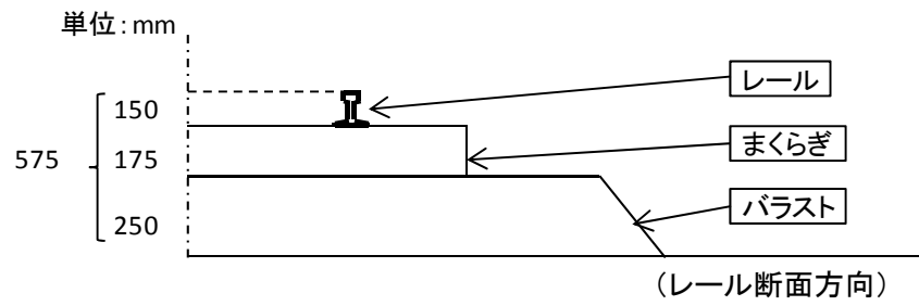
鉄道軌道断面図 (ヒアリング結果を基に水管理・国土保全局が作成)
