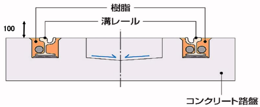
路面電車・LRT 軌道断面図 (LRT都市サミット広島 2009_鉄道局講演資料 91) )
