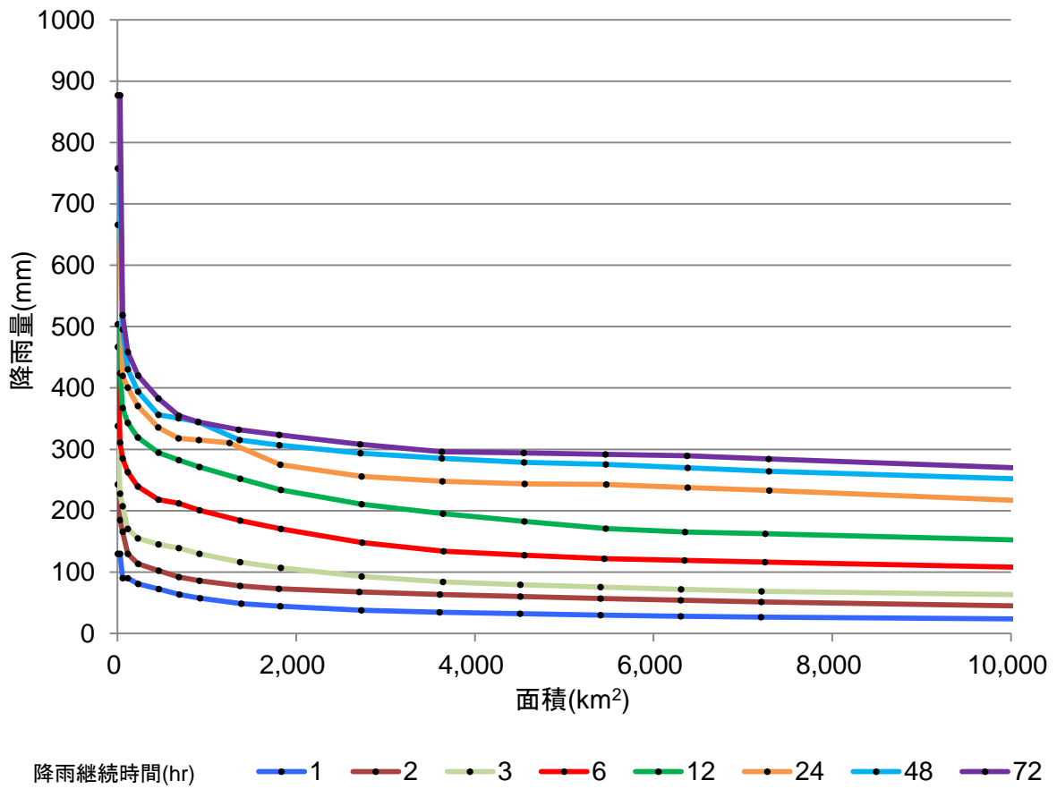
別添図-2 実績最大降雨量の包絡線 (②北海道南部)
