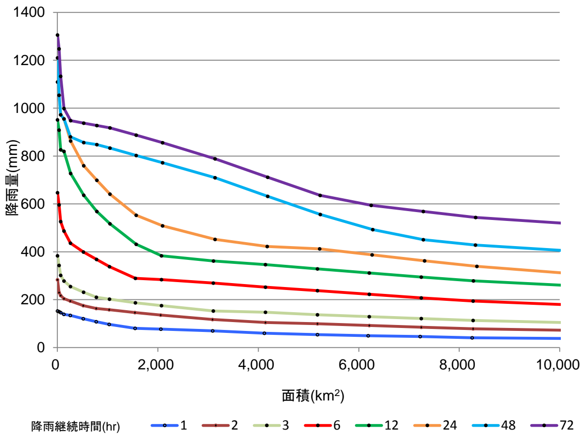
別添図-14 実績最大降雨量の包絡線 (⑭九州北西部)
