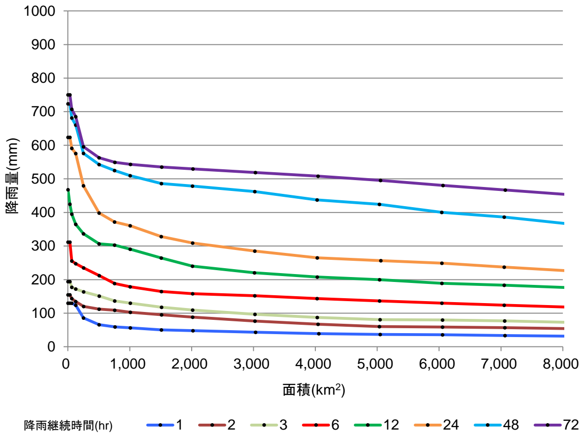
別添図-10 実績最大降雨量の包絡線 (⑩山陰)
