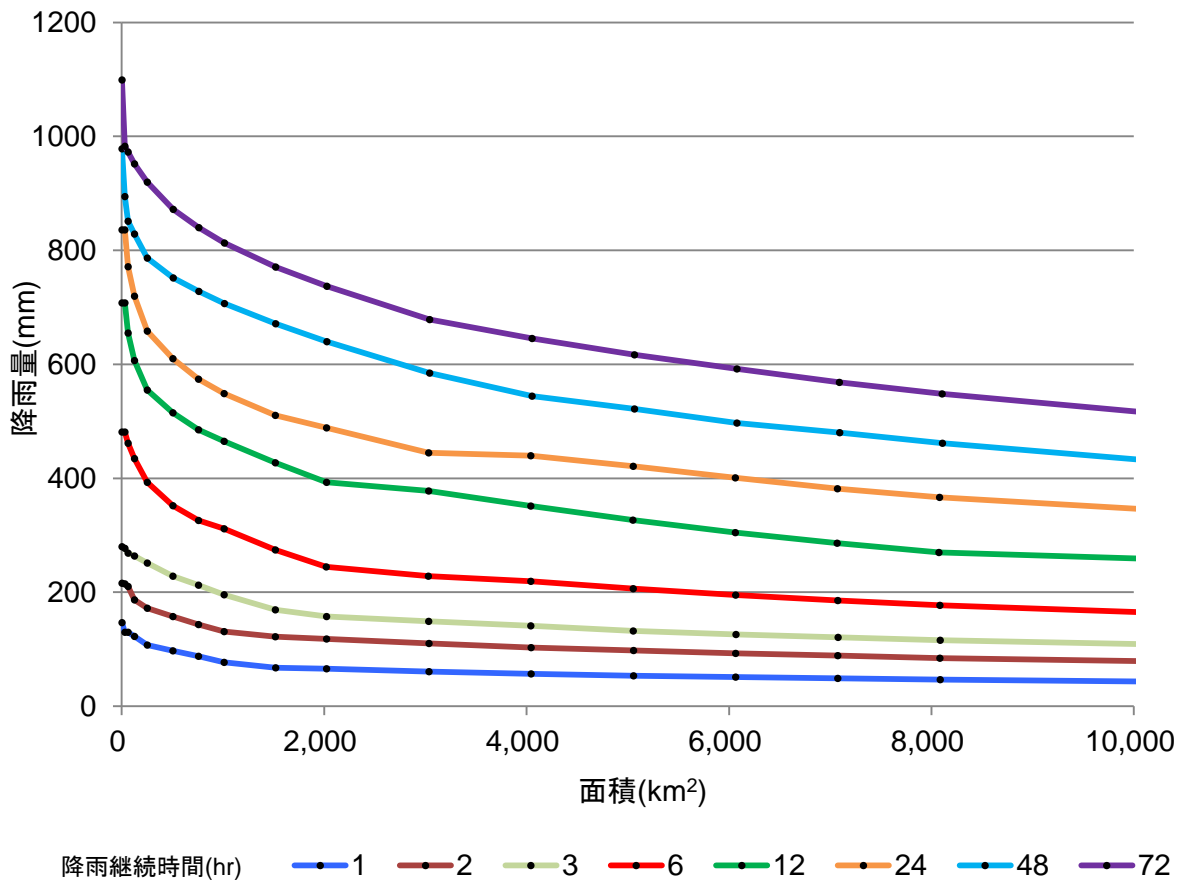
別添図-7 実績最大降雨量の包絡線 (⑦中部)
