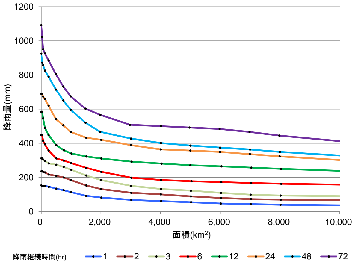
別添図-5 実績最大降雨量の包絡線 (⑤ 関東)
