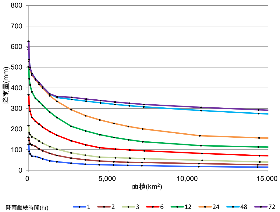
別添図-1 実績最大降雨量の包絡線 (①北海道北部)
