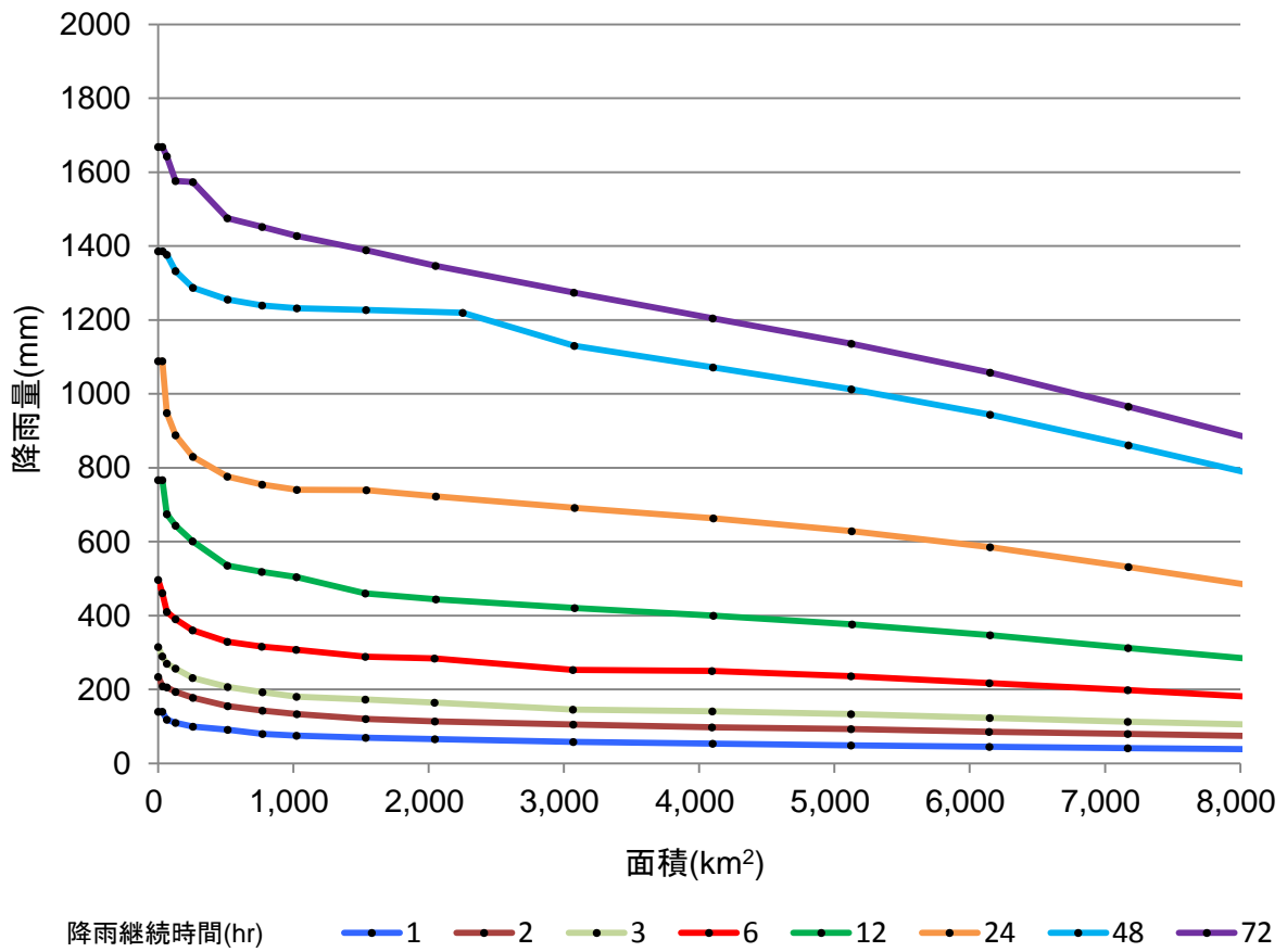
別添図-9 実績最大降雨量の包絡線 (⑨紀伊南部)
