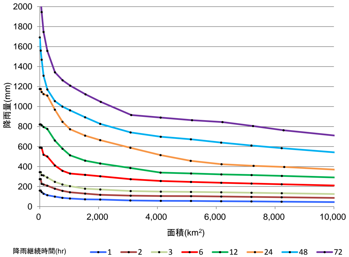
別添図-13 実績最大降雨量の包絡線 (⑬四国南部)
