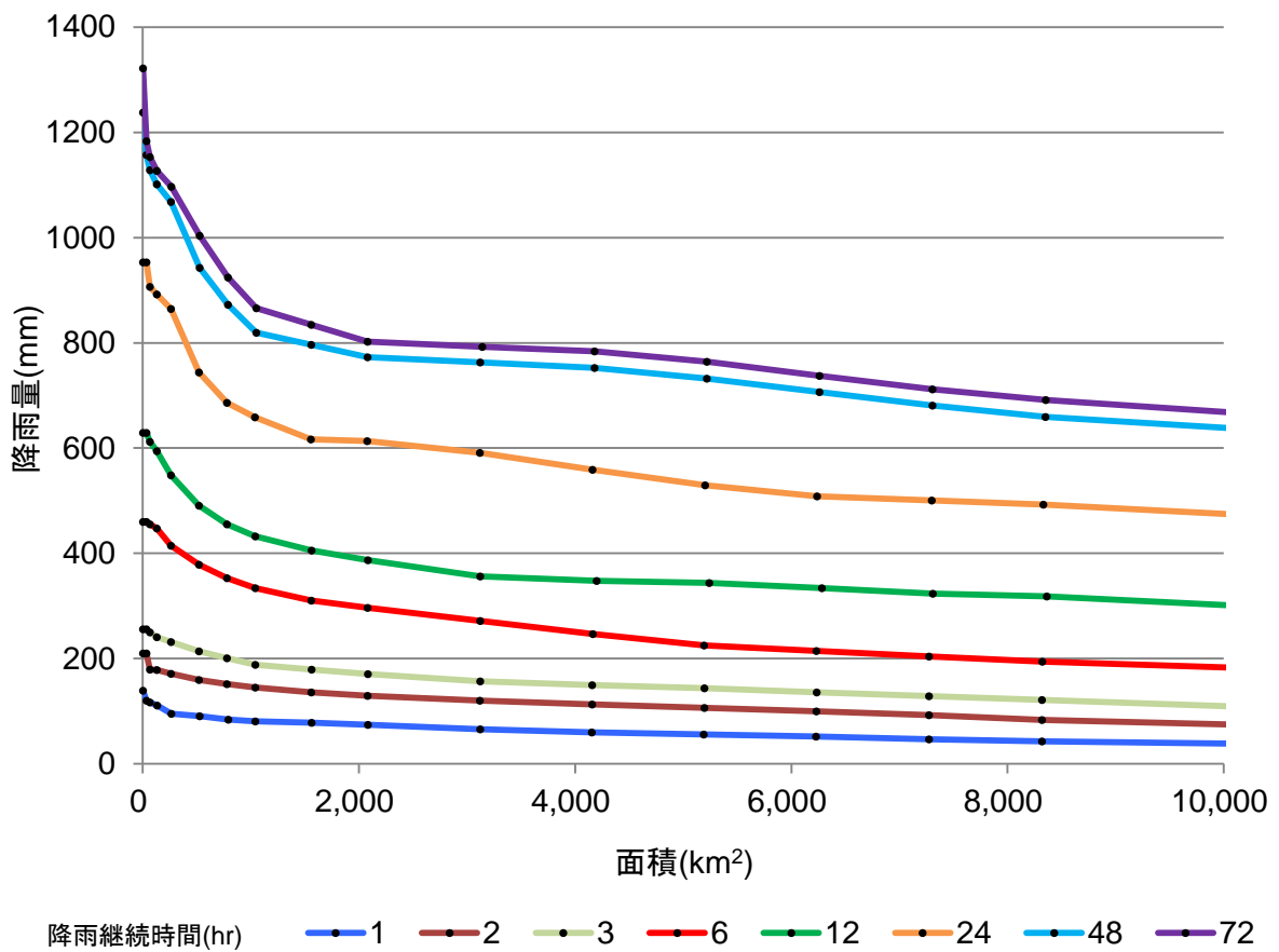
別添図-15 実績最大降雨量の包絡線 (⑮九州南東部)
