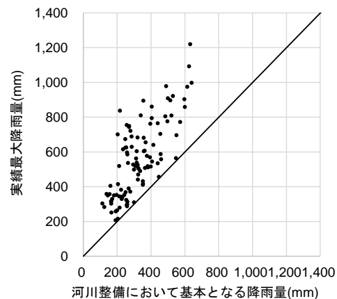
図-3 一級水系における実績最大降雨量と河川整備において基本となる降雨量
