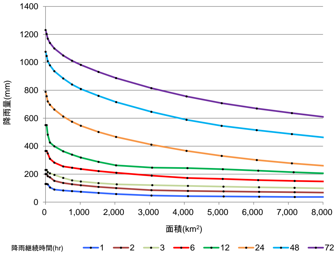
別添図-11 実績最大降雨量の包絡線 (⑪瀬戸内)
