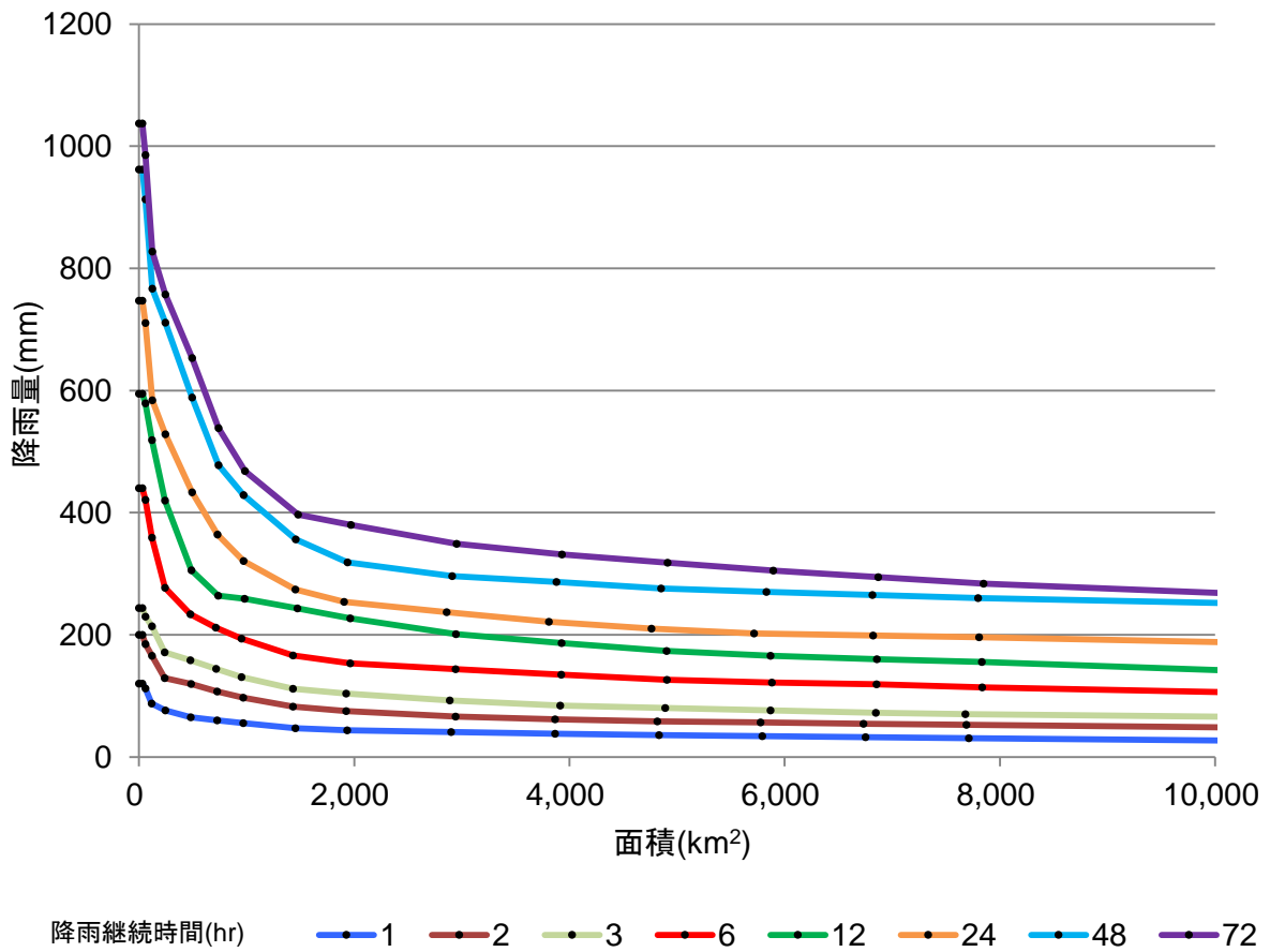
別添図-4 実績最大降雨量の包絡線 (④東北東部)
