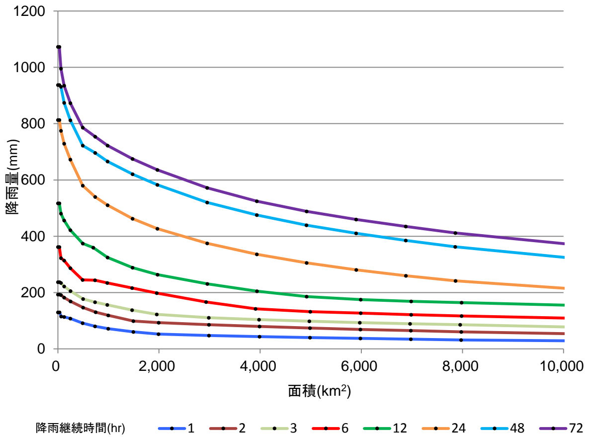
別添図-6 実績最大降雨量の包絡線 (⑥北陸)
