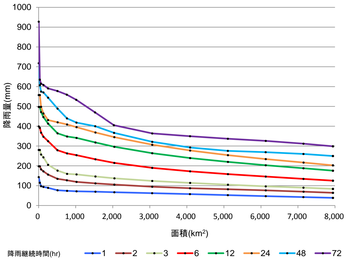
別添図-12 実績最大降雨量の包絡線 (⑫中国西部)
