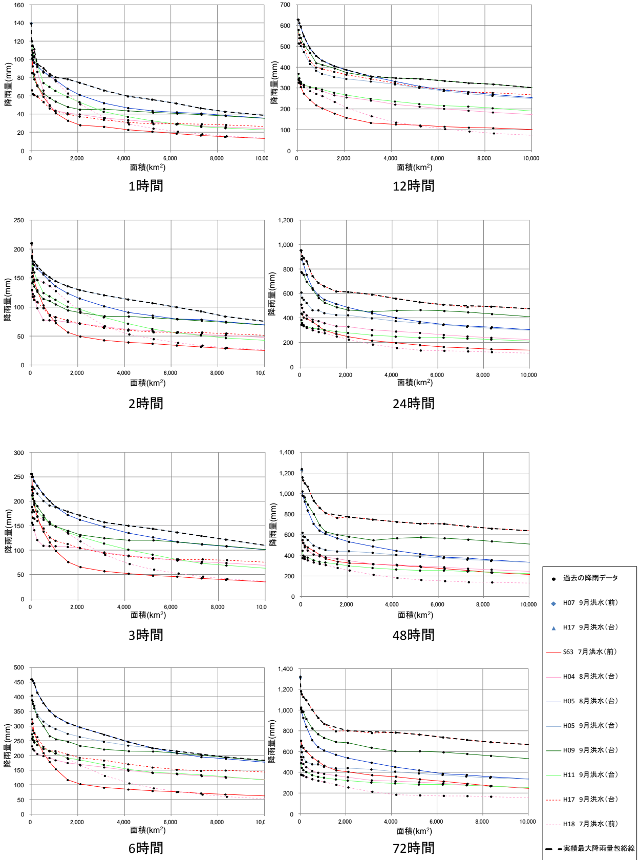
参考図 2-3(15) 実績最大降雨量と包絡線 (⑮九州南東部)
