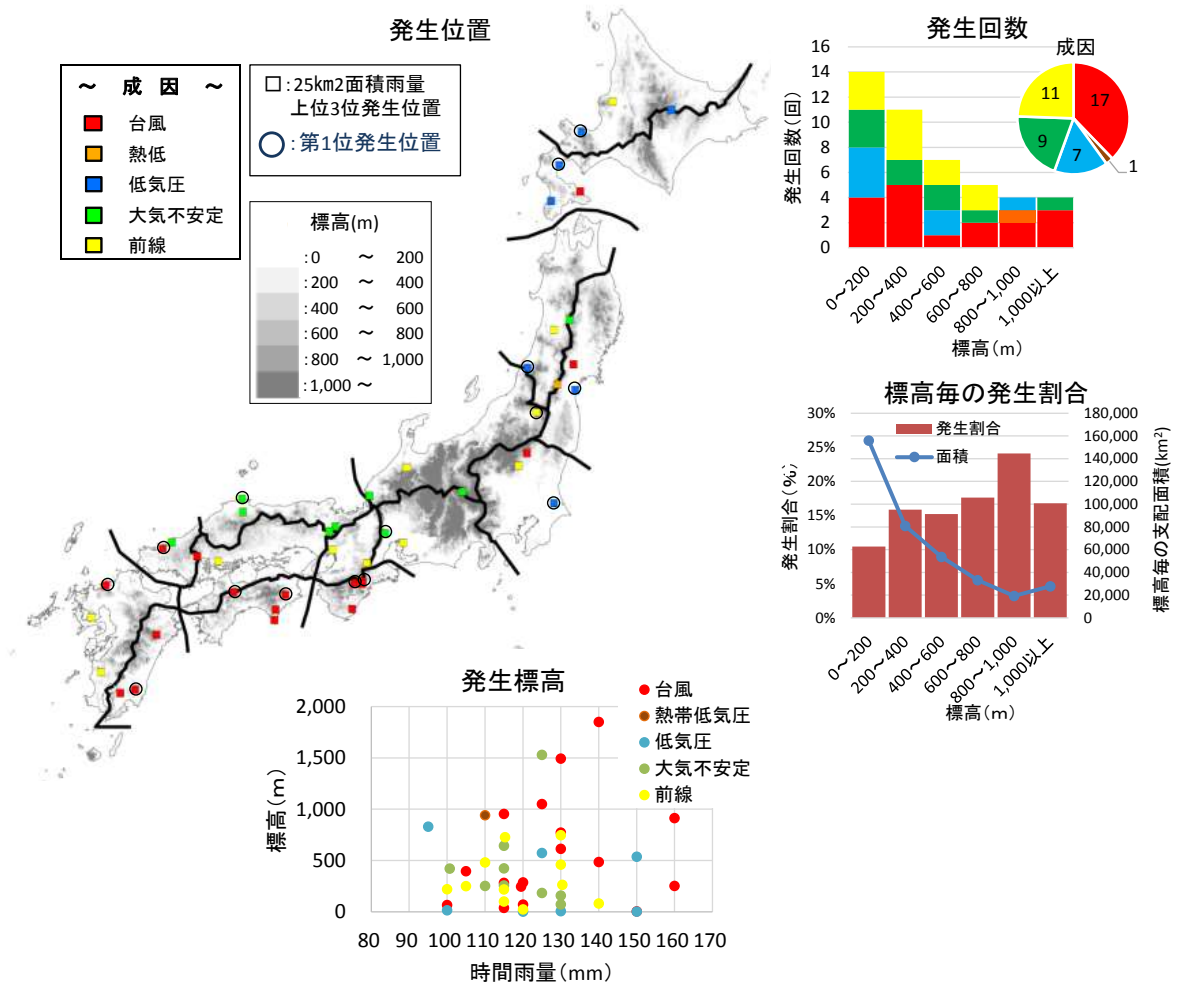
参考図 2-5 約 5km 四方データ (約 25km 2 ) の 1 時間降雨量 (上位 3 位) について
