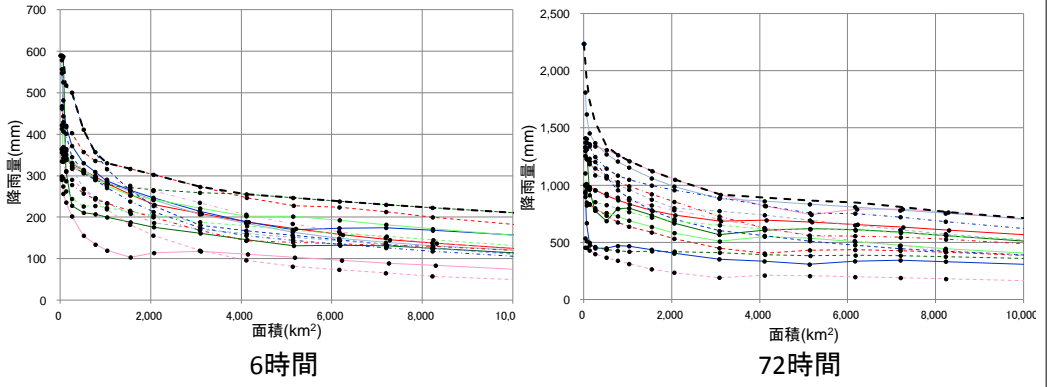
参考図 2-3(13) 実績最大降雨量と包絡線 (⑬四国南部)
