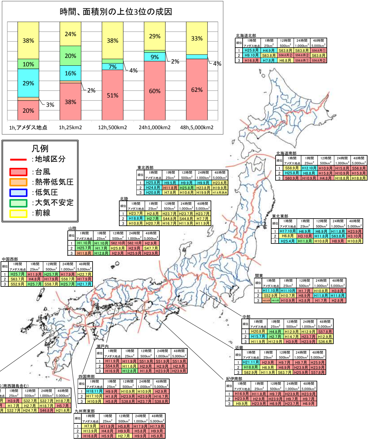
参考図 2-6 降雨継続時間別、面積別の降雨量の成因について
