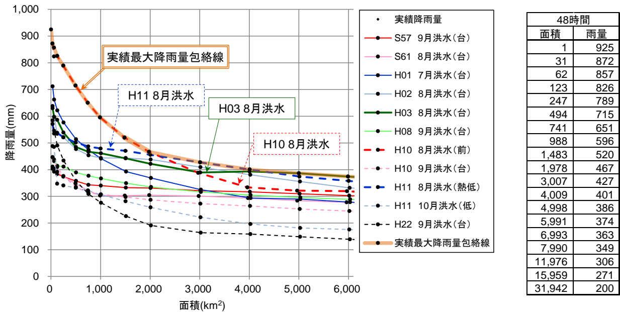
参考図 2-2 実績最大降雨量に関する解析と包絡線の作成（イメージ）
