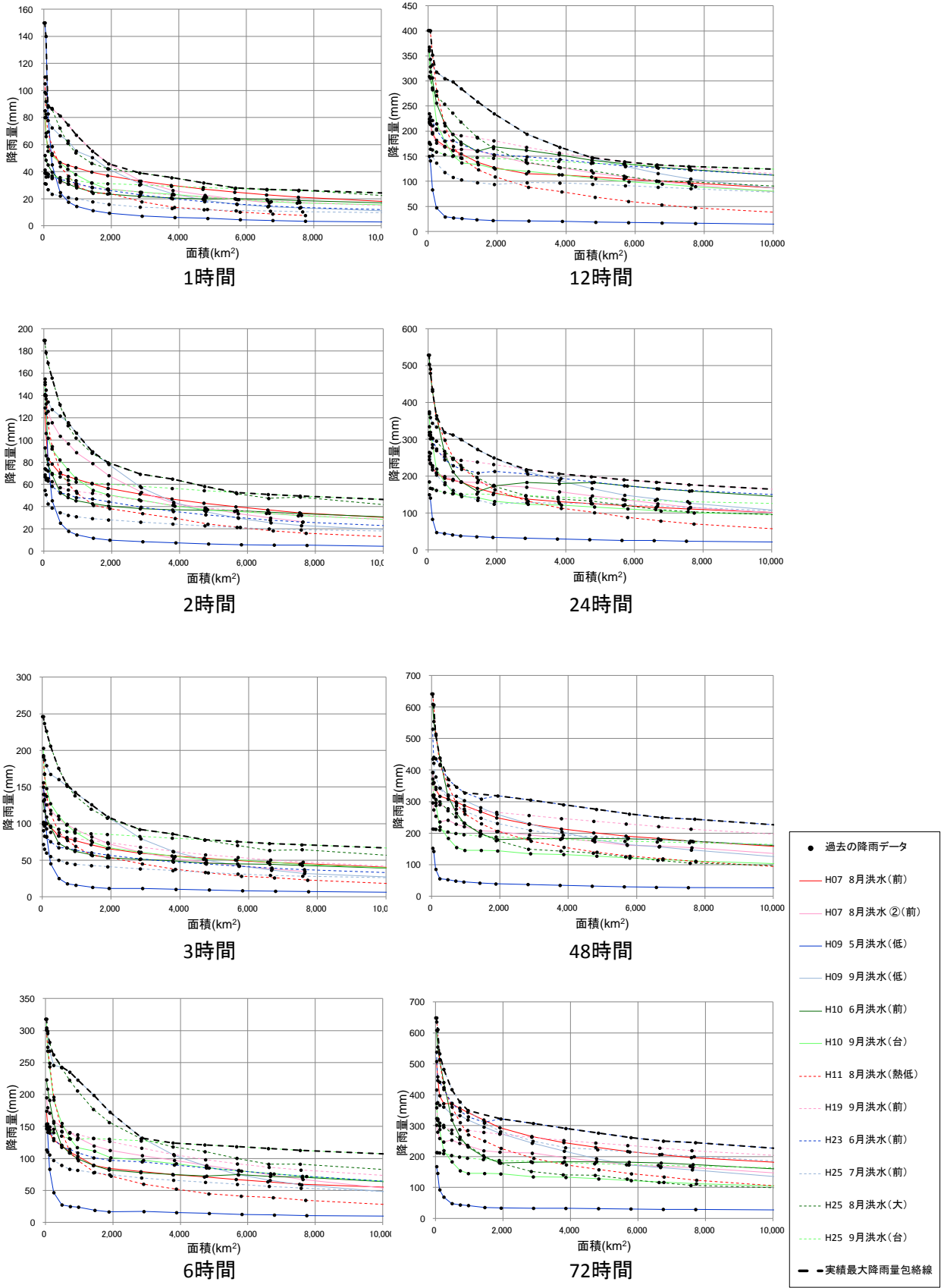
参考図 2-3(3) 実績最大降雨量と包絡線 (③東北西部)
