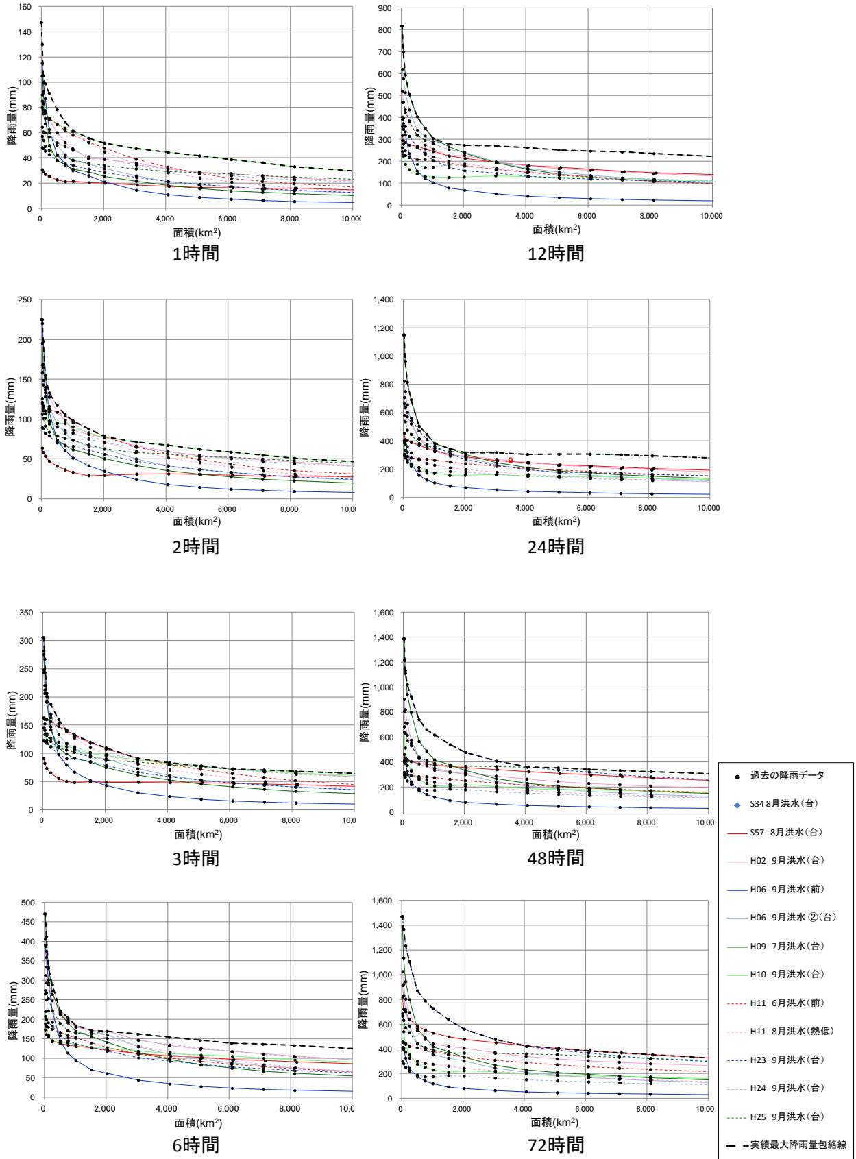
参考図 2-3(8) 実績最大降雨量と包絡線 (⑧近畿)
