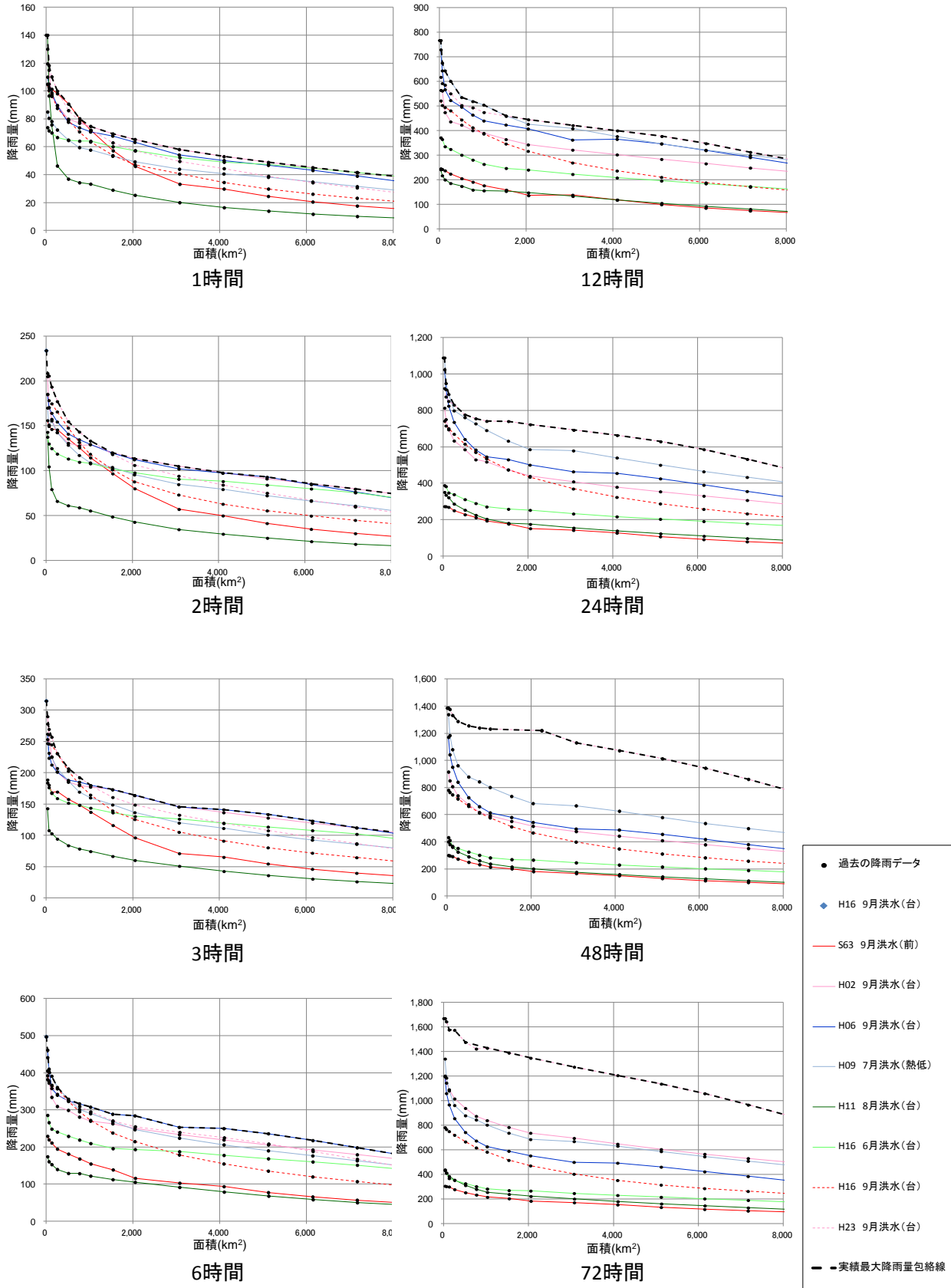
参考図 2-3(9) 実績最大降雨量と包絡線 (⑨紀伊南部)
