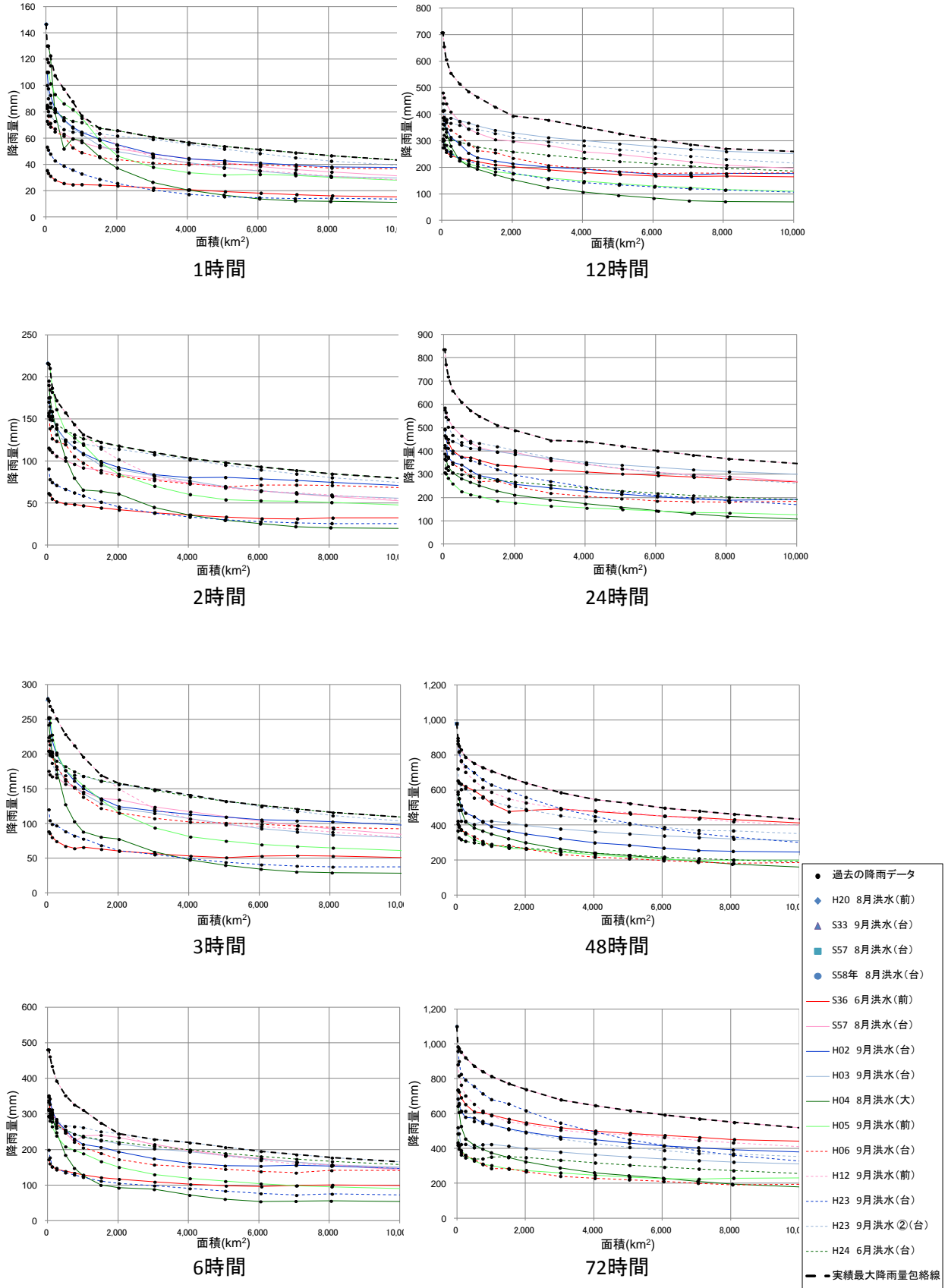
参考図 2-3(7) 実績最大降雨量と包絡線 (⑦中部)
