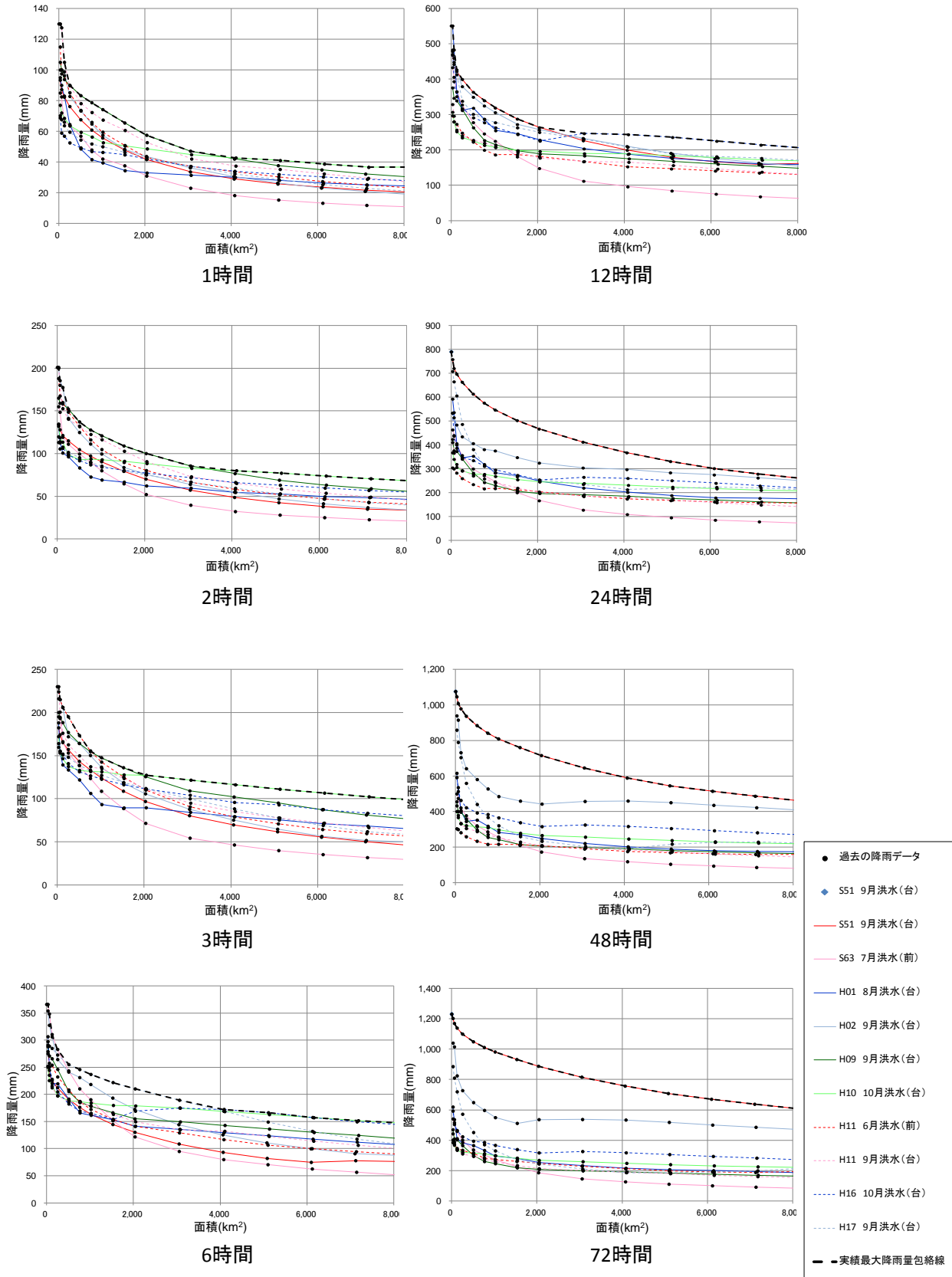
参考図 2-3(11) 実績最大降雨量と包絡線 (①瀬戸内)
