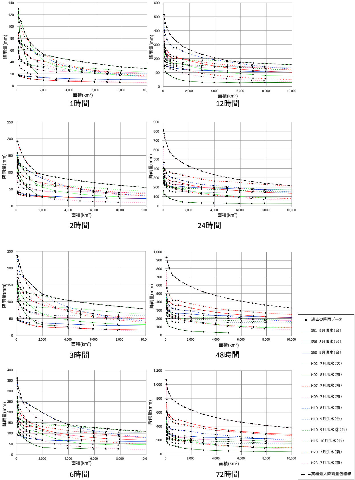
参考図 2-3(6) 実績最大降雨量と包絡線 (⑥北陸)
