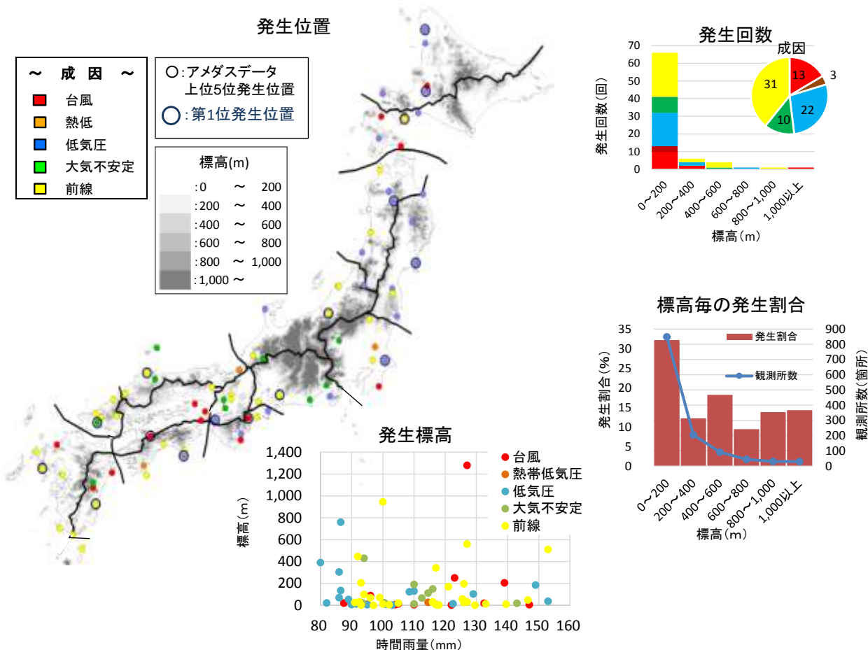
参考図 2-4 アメダスデータの 1 時間降雨量（上位 5 位）について
