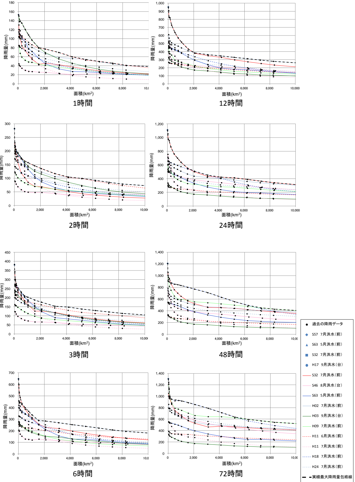
参考図 2-3(14) 実績最大降雨量と包絡線 (⑭九州北西部)
