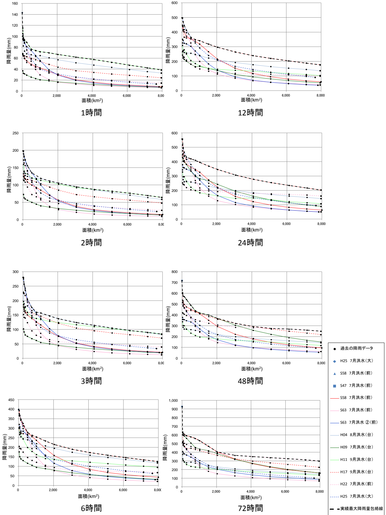
参考図 2-3(12) 実績最大降雨量と包絡線 (⑫中国西部)
