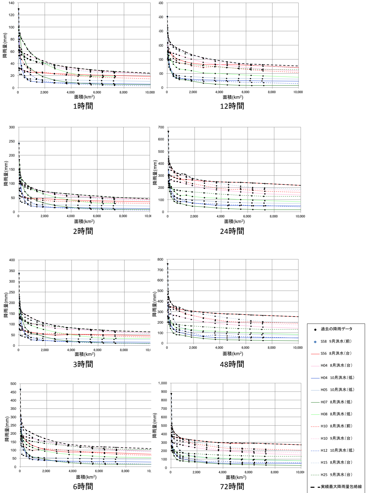
参考図 2-3(2) 実績最大降雨量と包絡線 (②北海道南部)
