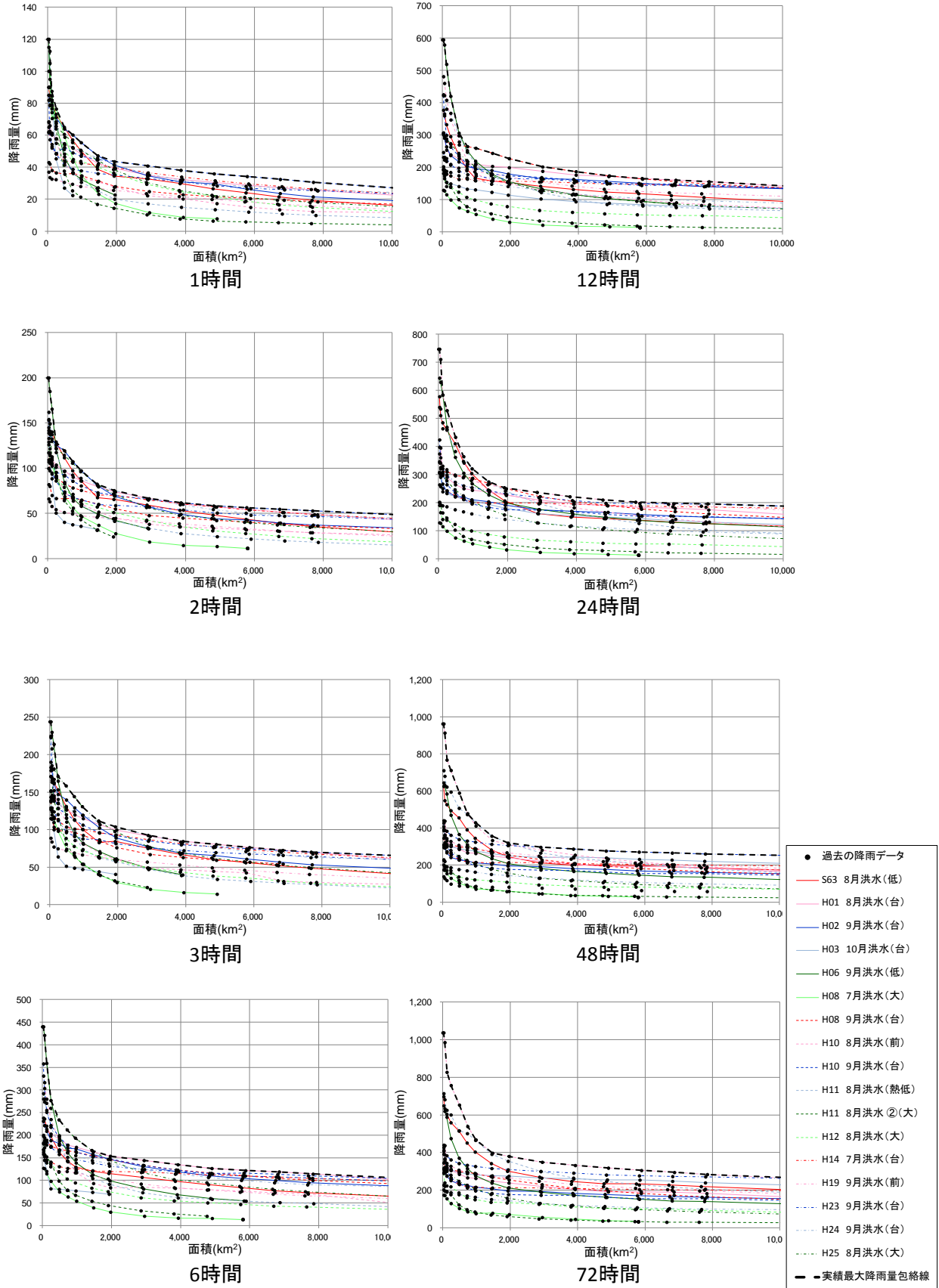
参考図 2-3(4) 実績最大降雨量と包絡線 (④東北東部)
