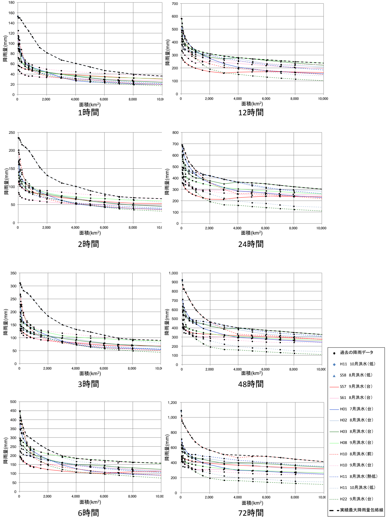
参考図 2-3(5) 実績最大降雨量と包絡線 (⑤関東)
