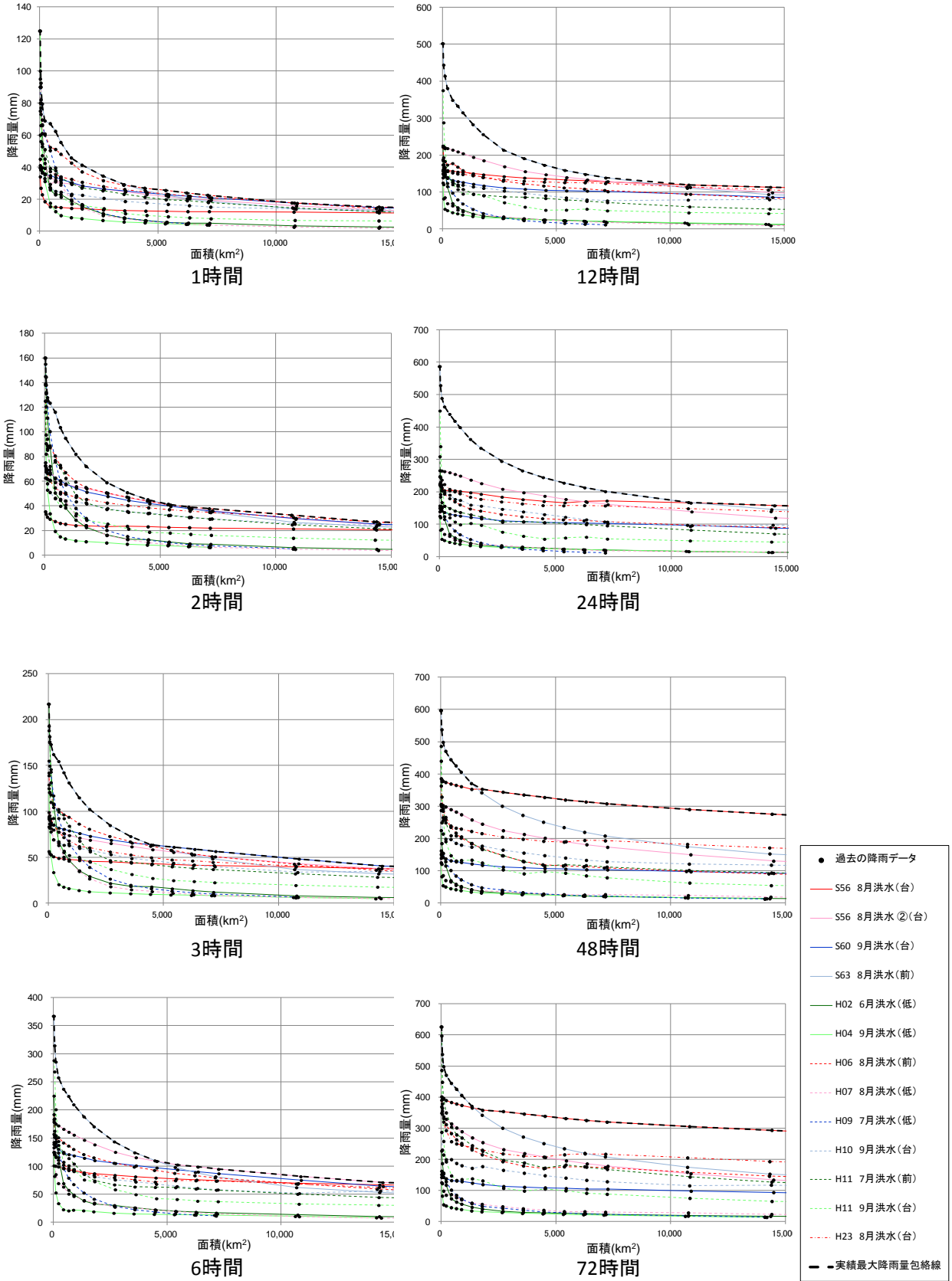
参考図 2-3(1) 実績最大降雨量と包絡線 (①北海道北部)
