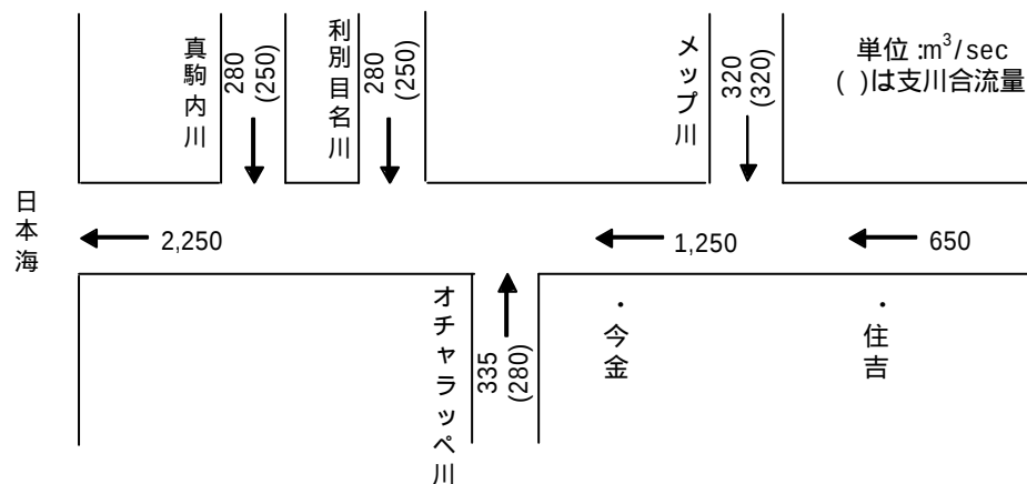
後志利別川計画高水流量図
