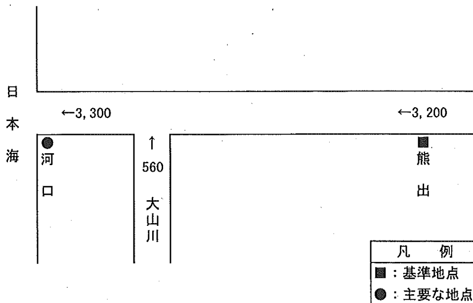
赤川計画高水流量図 (単位: \text{m}^3/\text{s} )
