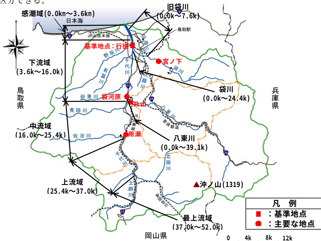
図 8.1.1 河道区分図
