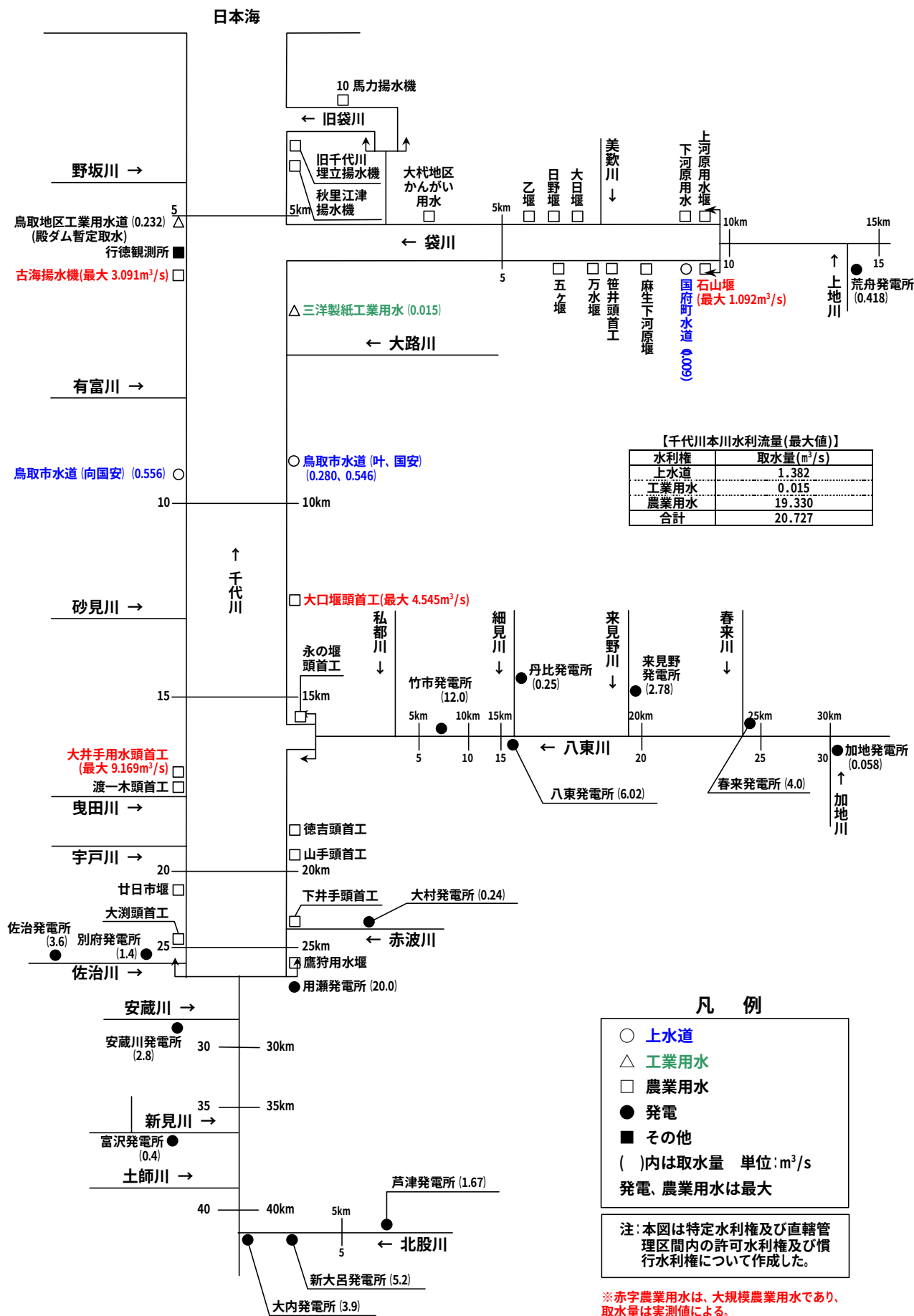
図 5.1.1 千代川水利権模式図
