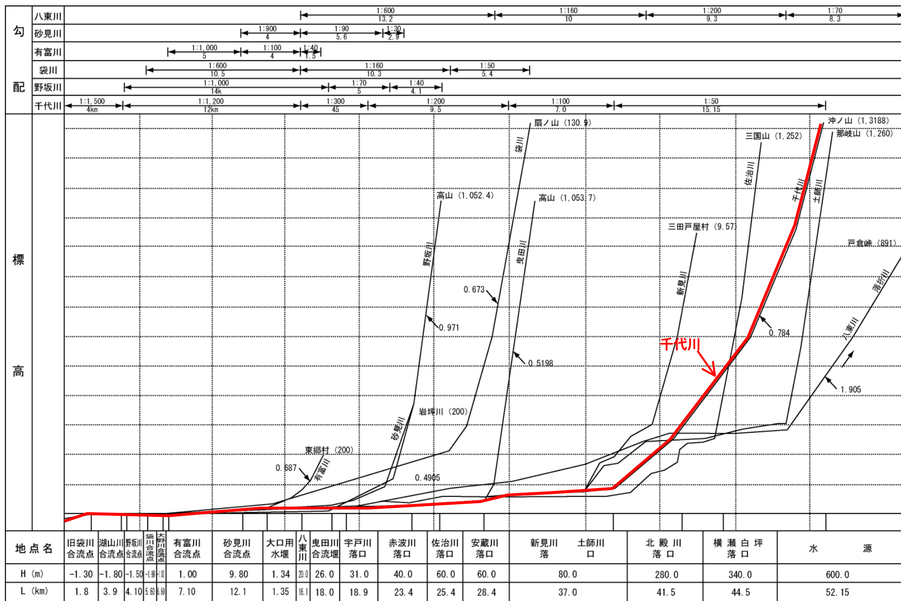
図 8.1.1 千代川水系河川縦断面図
