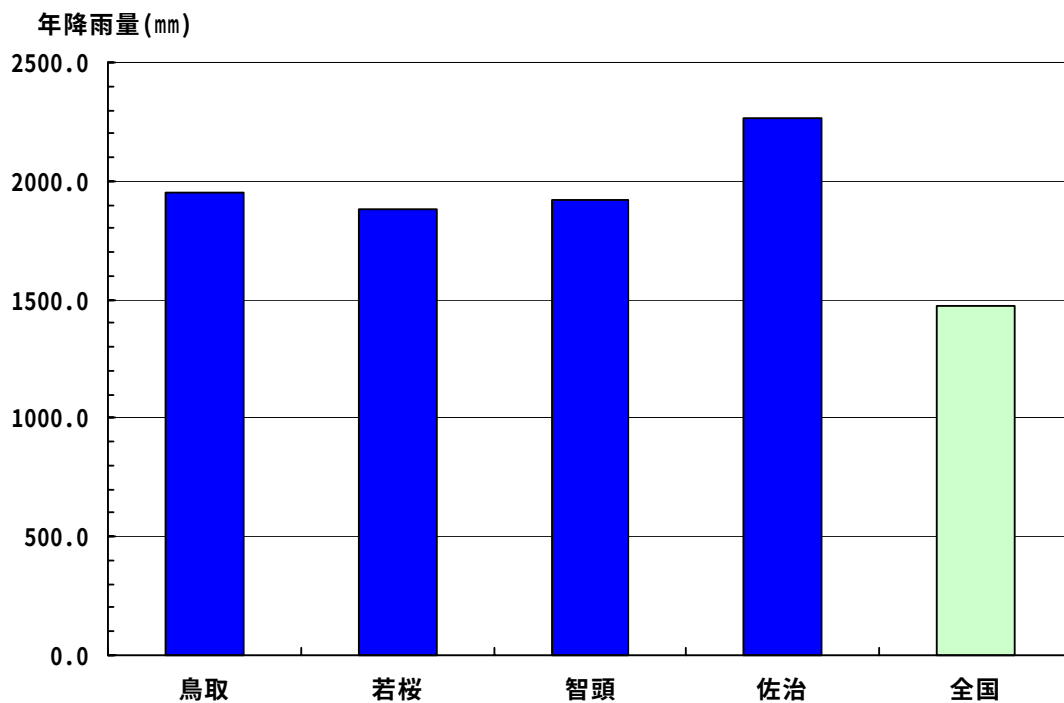
図 1.3.3 流域内の気象庁観測地点の年間平均降水量
