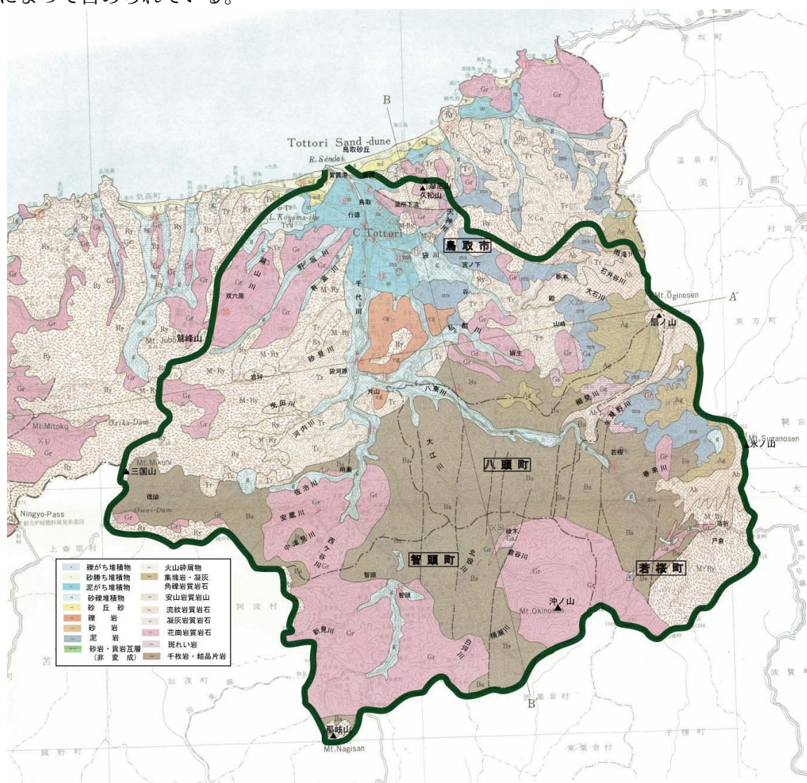
図 1.3.1 地質図
