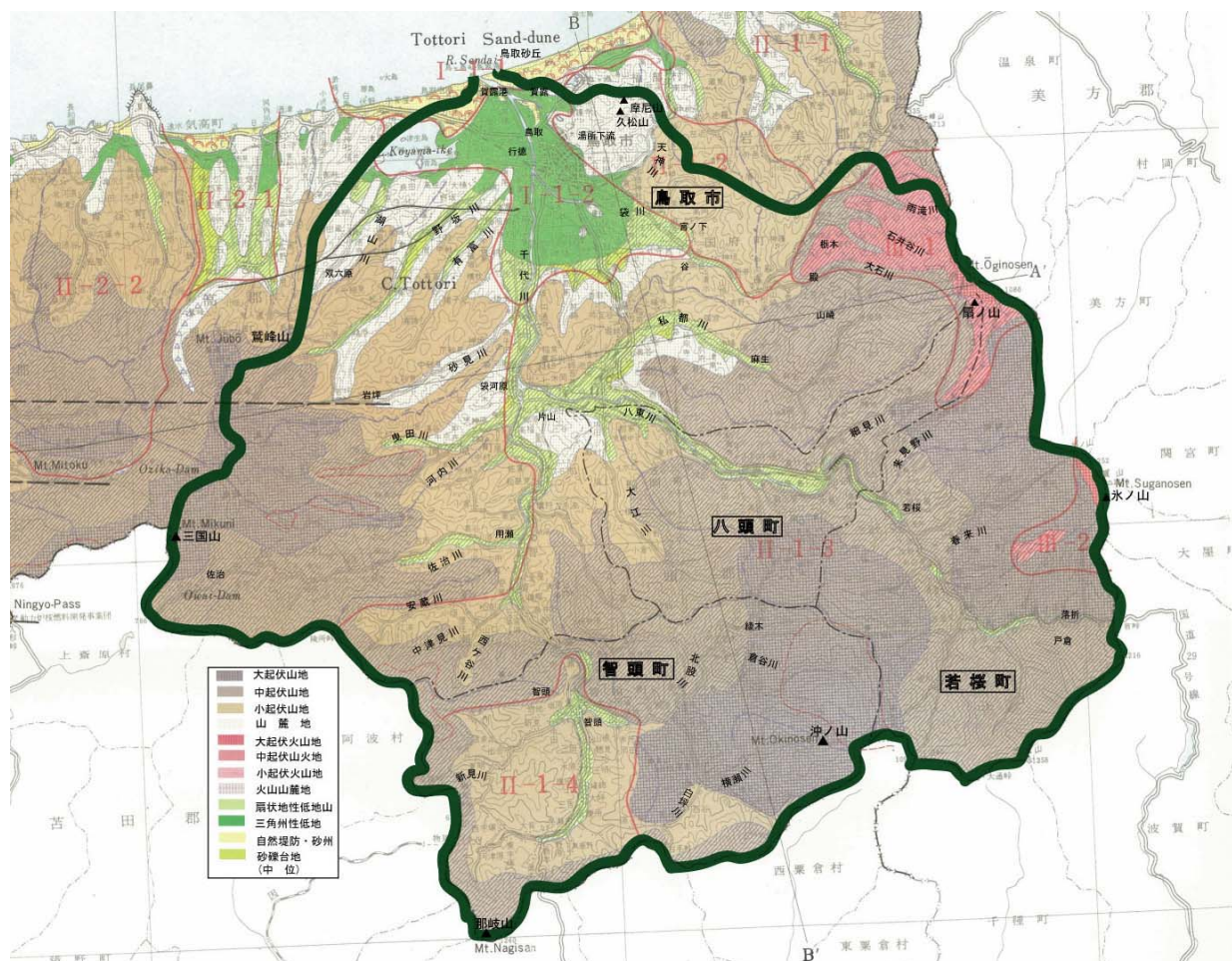
图 1.2.1 地形图
