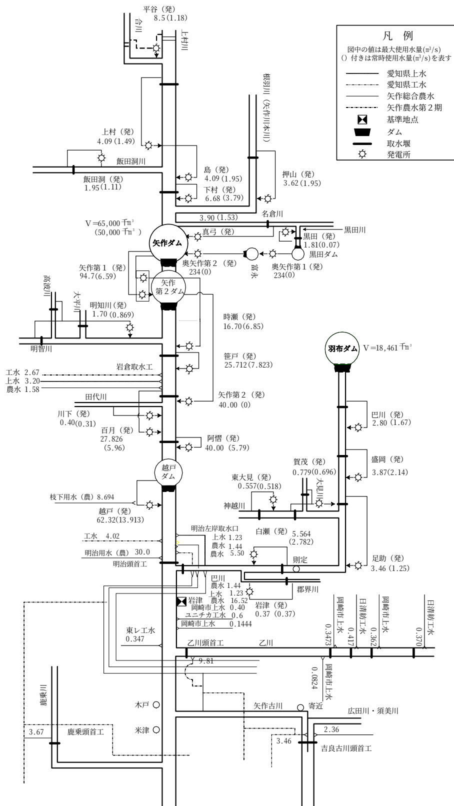
図 2-2 矢作川水系 水利使用模式図 (主要な水利権を記載)
