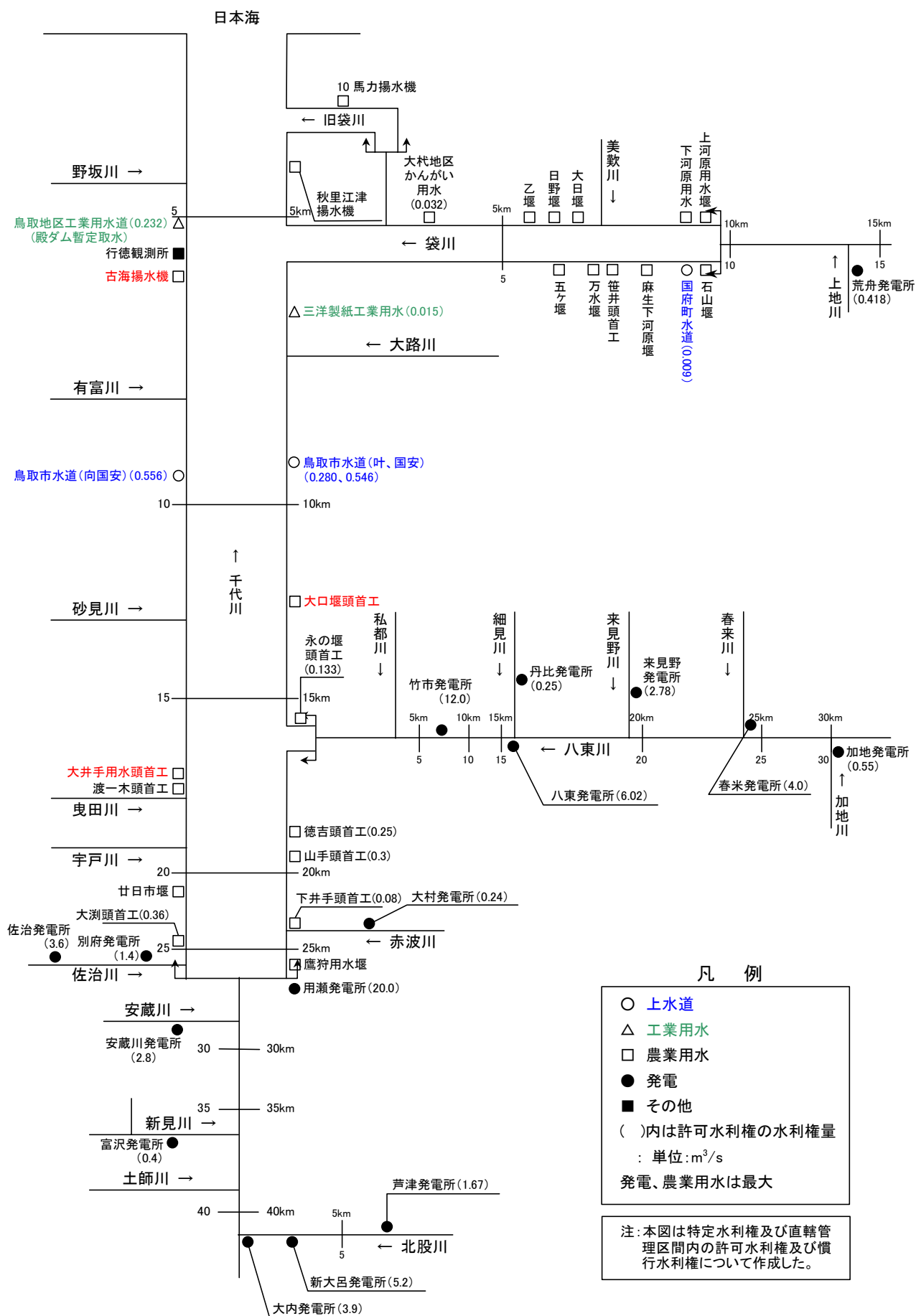
図 2-2 千代川水系の主な水利模式図
